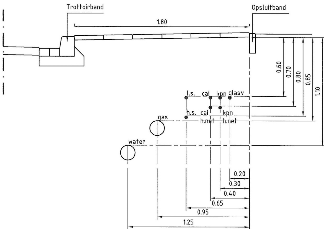
DWARSPROFIEL T.B.V. KABELS EN LEIDINGEN
