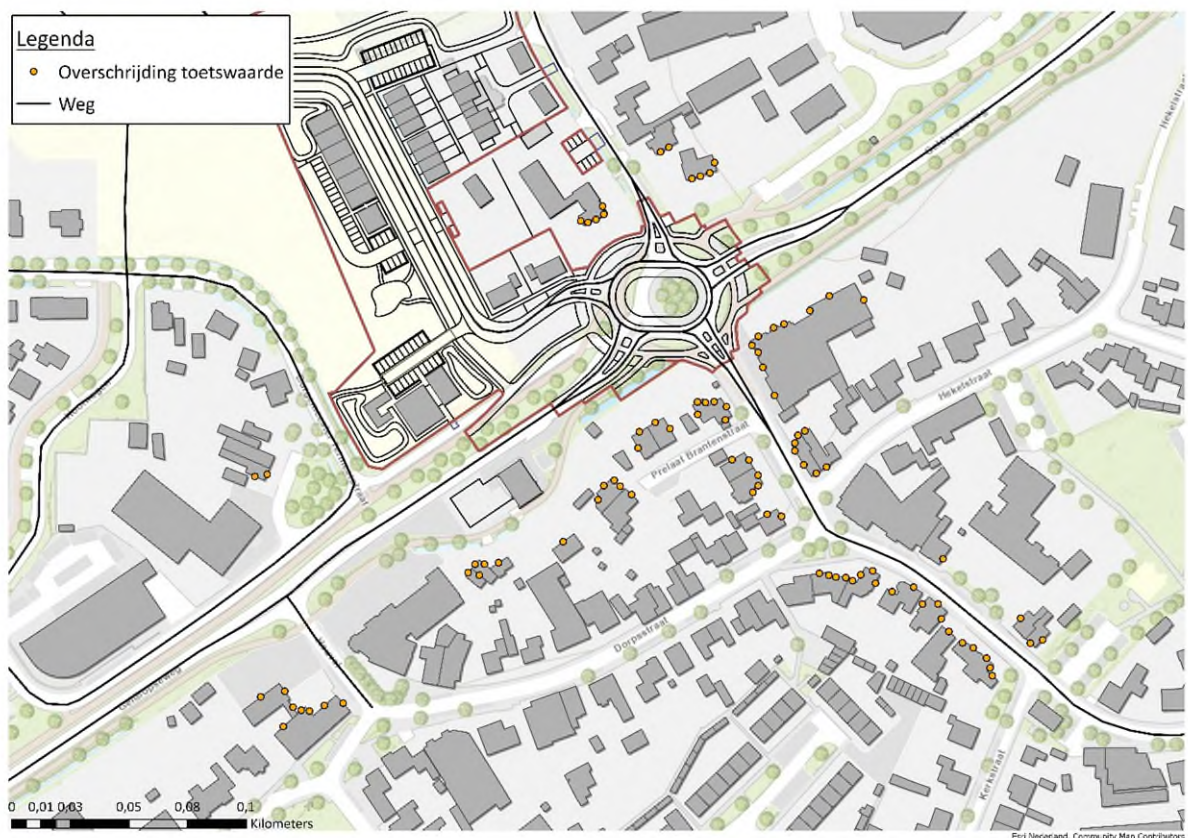
Figuur 4.1 Rekenpunten waar sprake is van een overschrijding van de toetswaarde als gevolg van de wijziging.
