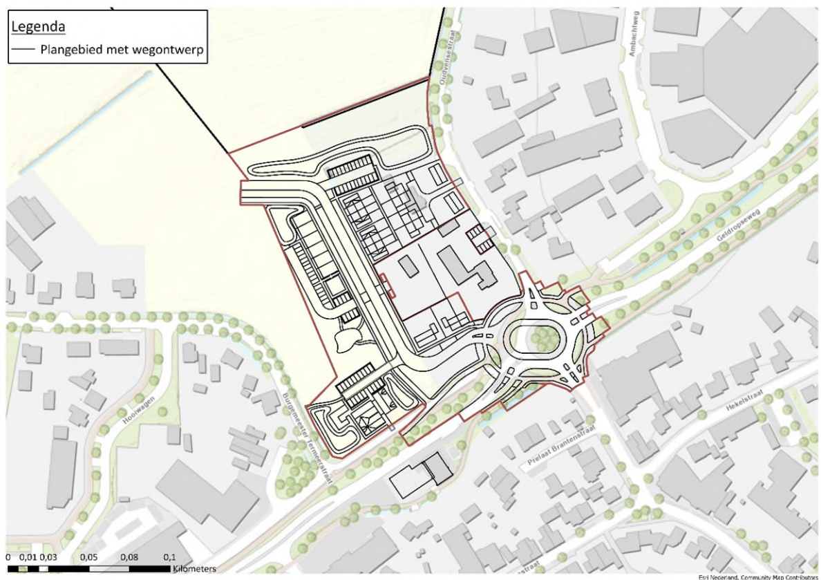
Figuur 1.1 Weergave van het plangebied en wegontwerp voor de wijziging aan de weg bij Oudvensestraat-Zuid.
