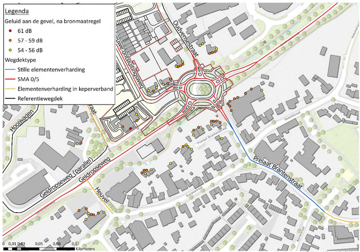
Figuur 5.2 Locaties met een overschrijding van de toetswaarde of standaardwaarde, na toepassing van stille elementenverharding op de Prelaat Brantenstraat en SMA 0/5 op de nieuwe ontsluitingsweg.
