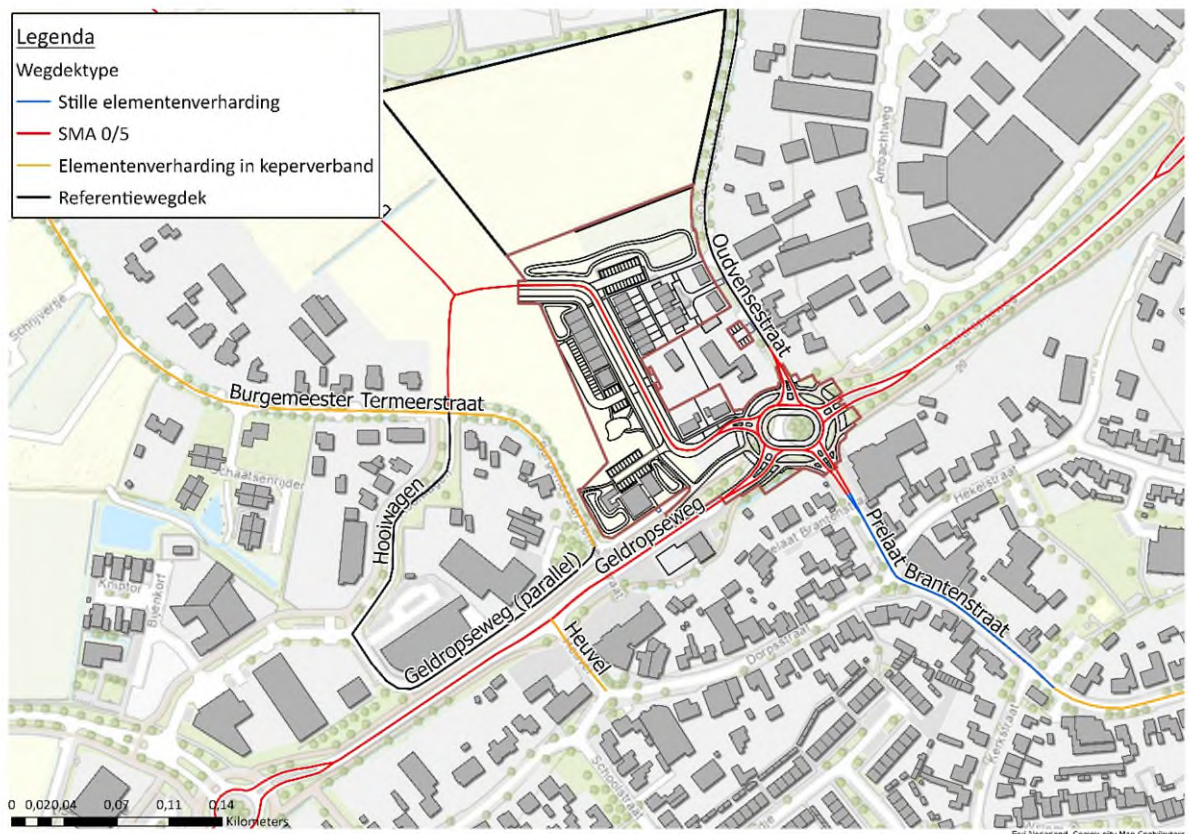
Figuur 5.1 Ligging van wegdektypes na toepassing van mogelijke geluidmaatregelen.
