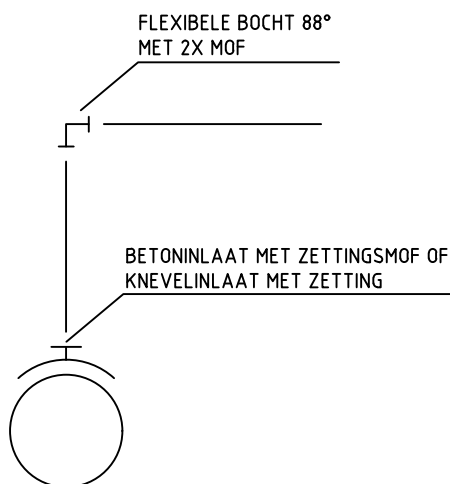
ENKELE KOLK- / HUISAANSLUITING
