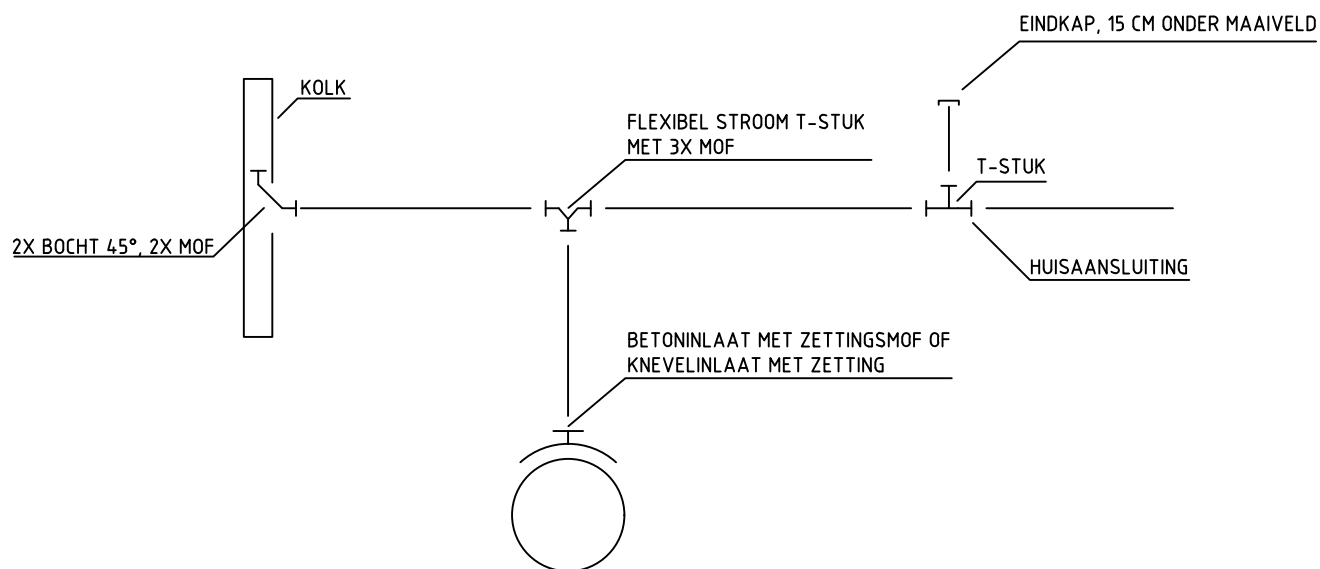
DUBBELE KOLK- / HUISAANSLUITING
