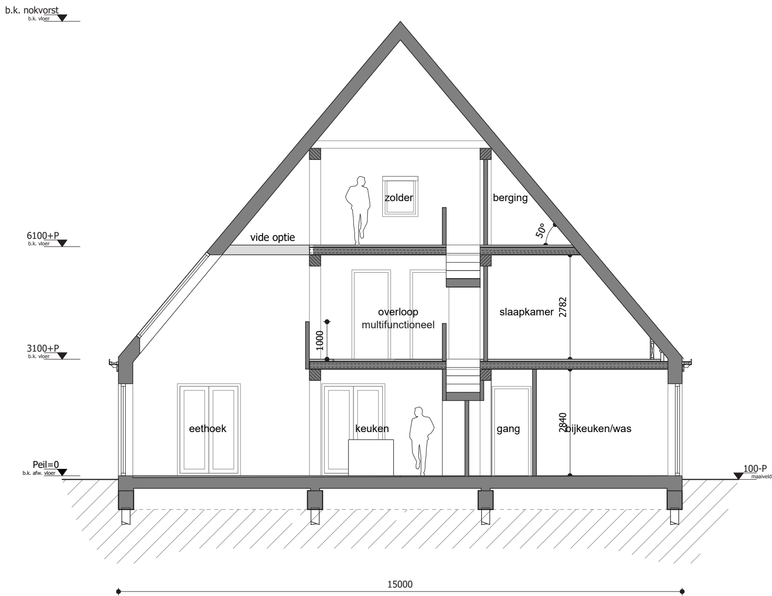
Doorsnede A-A
