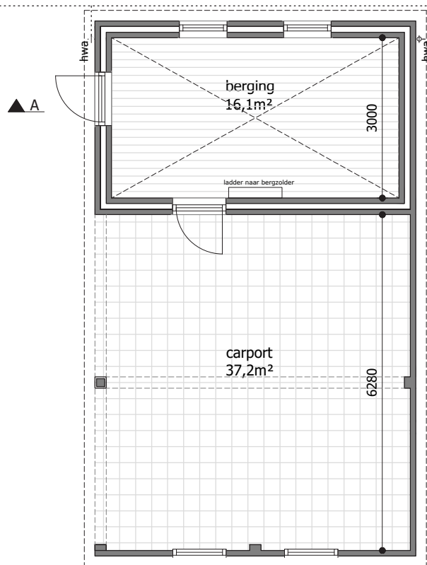
Begane grond
