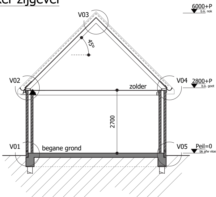
Doorsnede A-A
