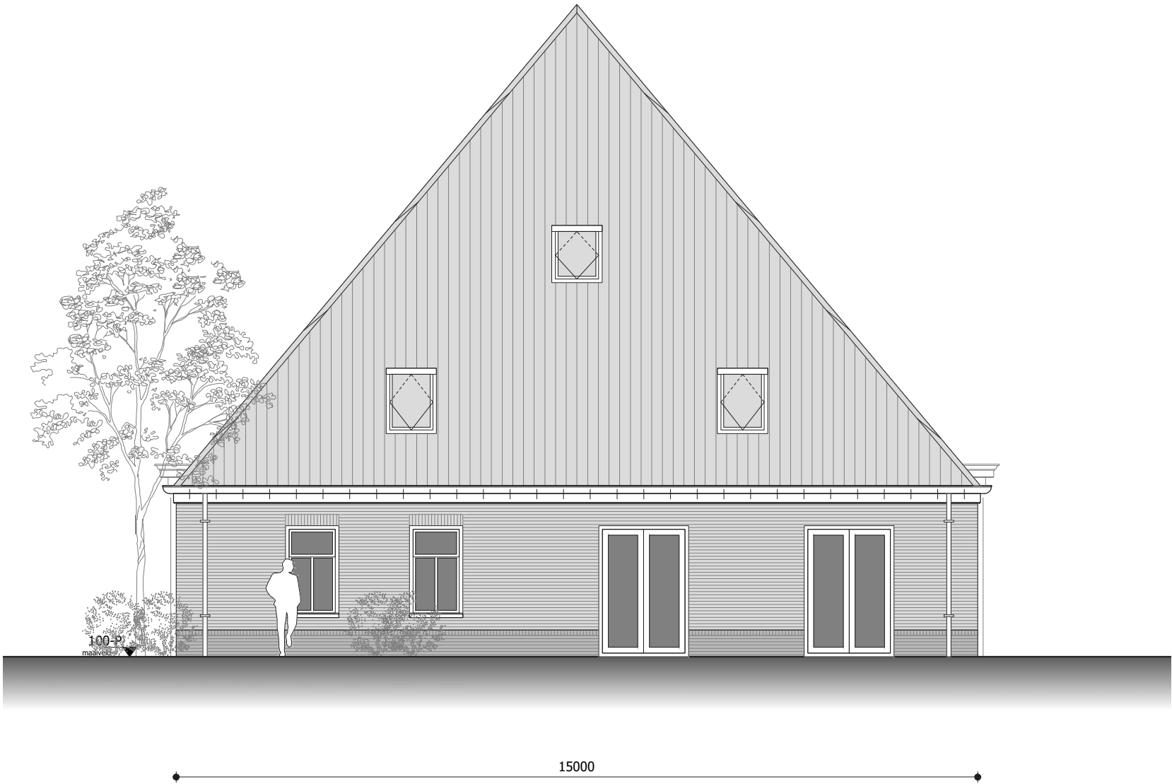
Achtergevel (west)
