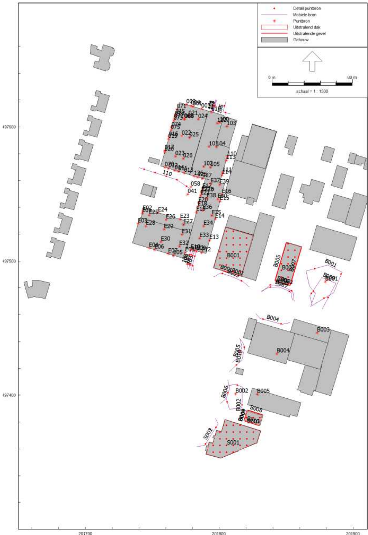
Figuur 2.2: Invoerplot rekenmodel – bronnen langtijdgemiddelde beoordelingsniveaus
