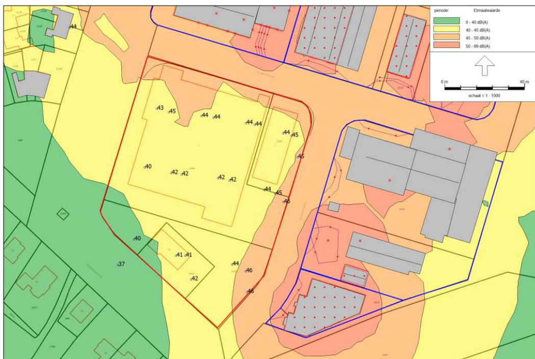
f3.2 Geluidcontouren (etmaalwaarde op 5m hoogte) uitgaande van een reële inschatting
