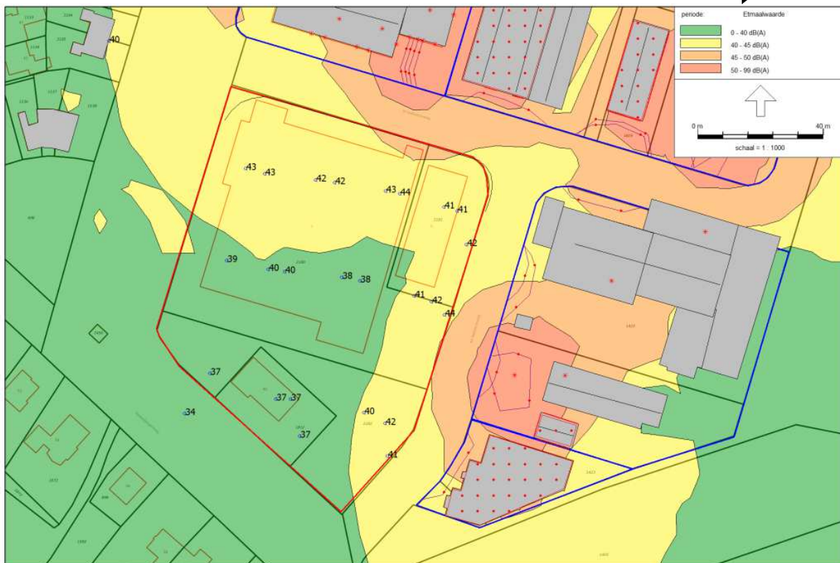
Figuur 3: Geluidcontouren verschillende hoogten
