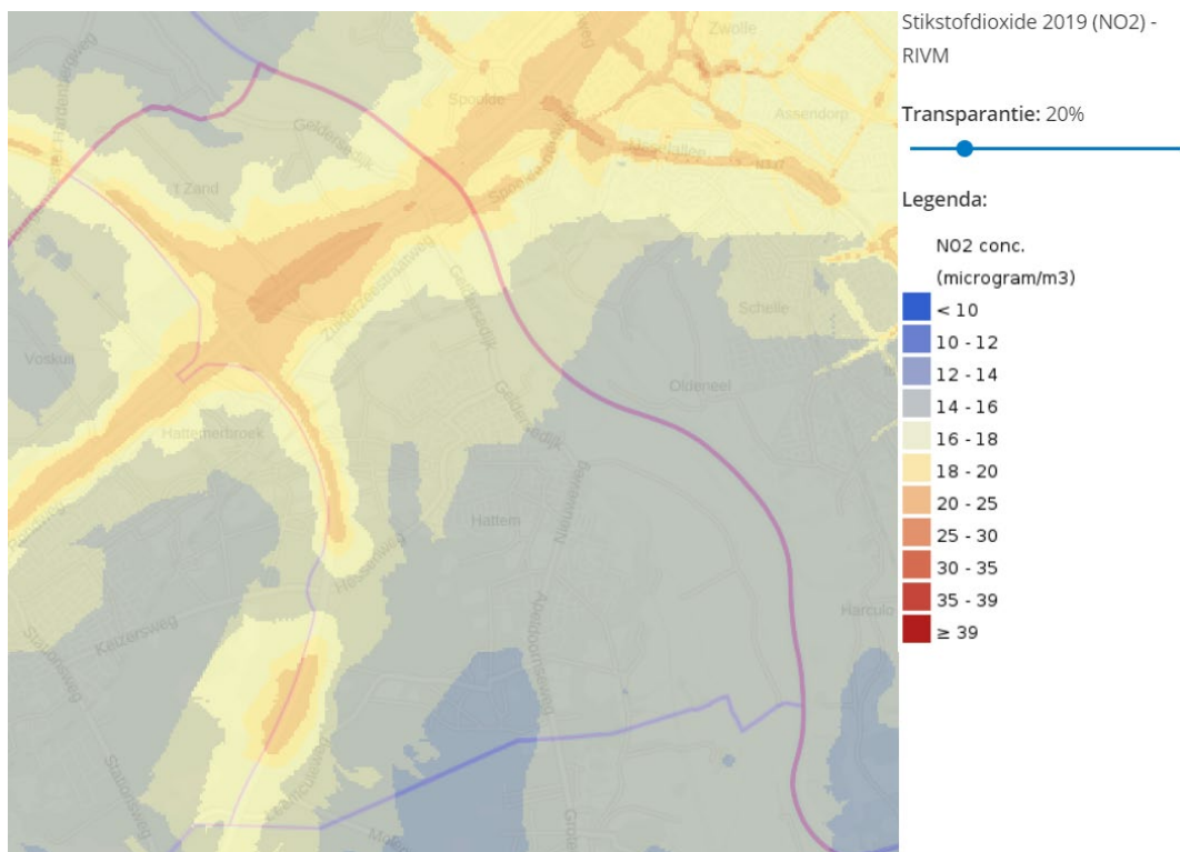
Figuur 4-5 Stikstofdioxide
