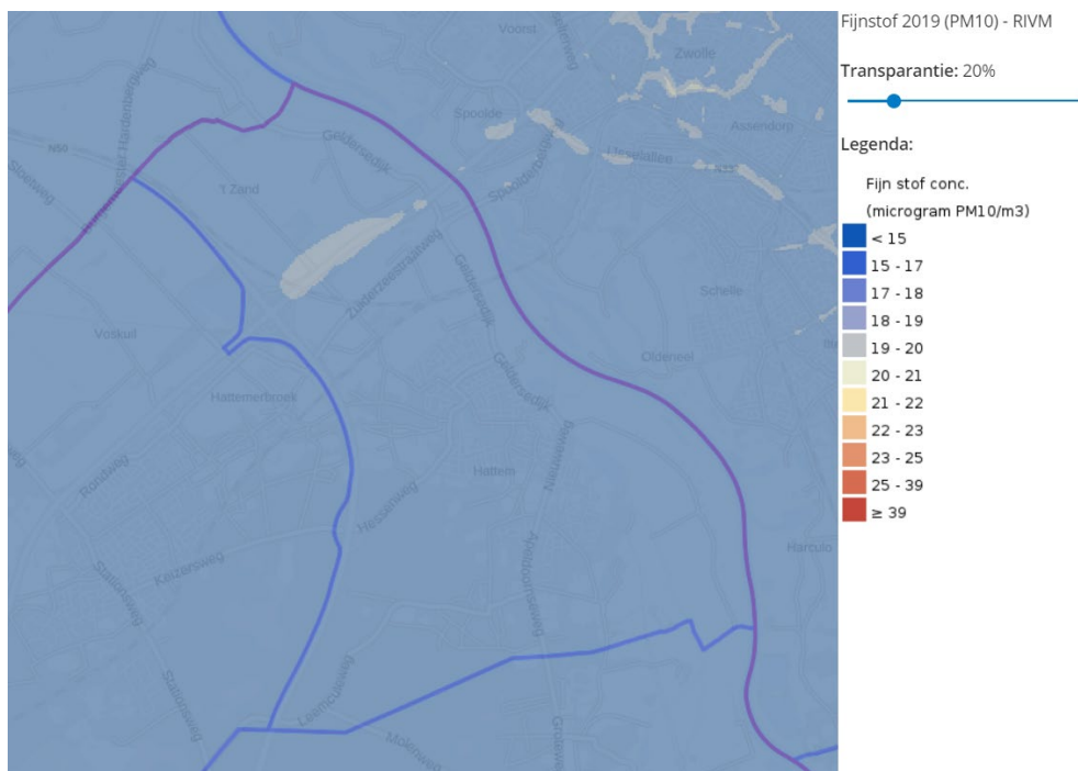
Figuur 4-7 Fijnstof PM10
