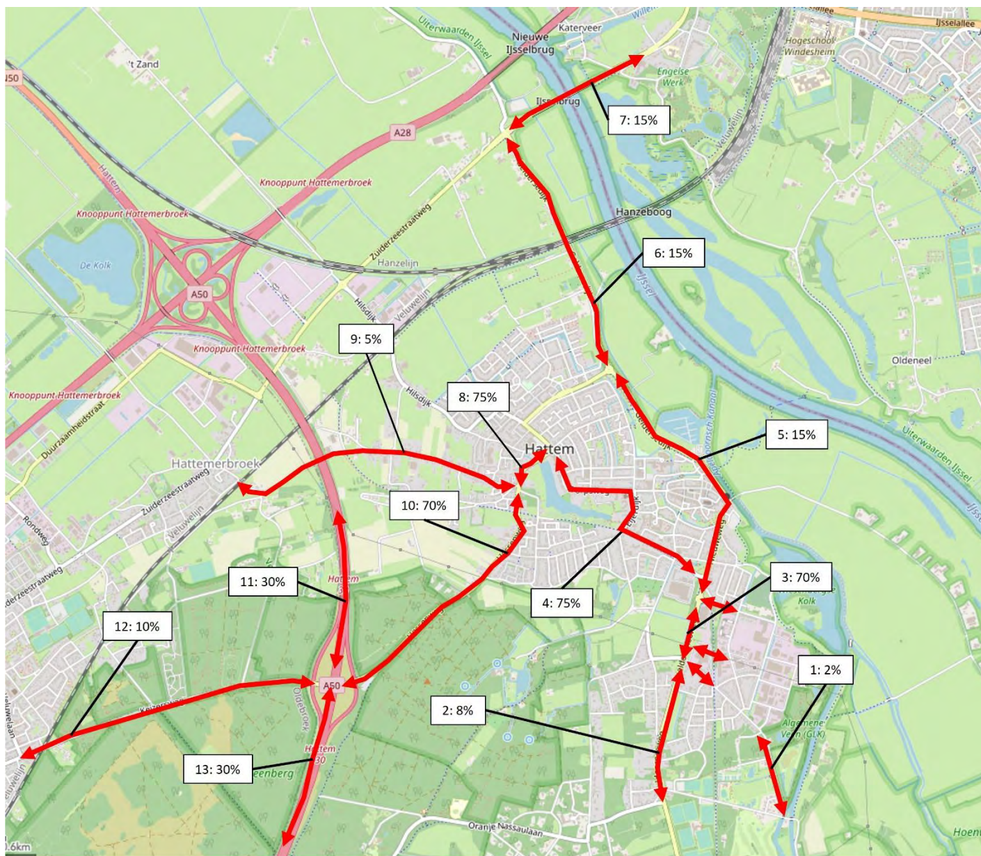
Figuur 2 De verkeerstoedeling beoogde ontwikkeling
