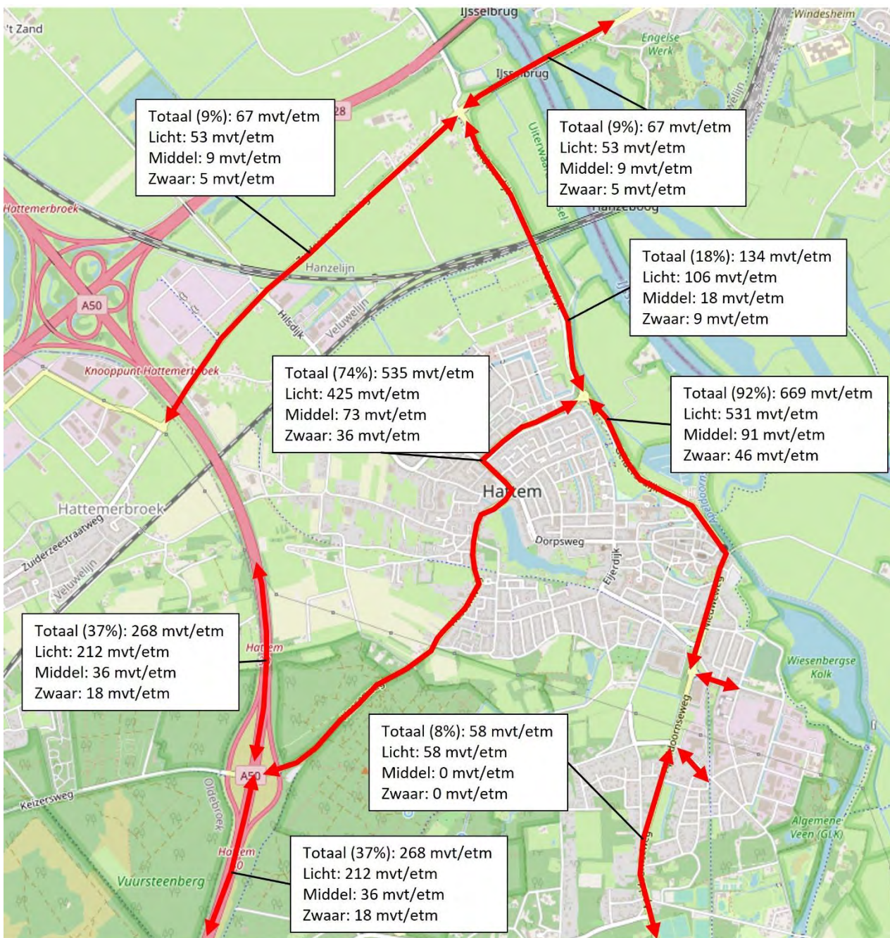
Figuur 1 de verkeerstoedeling van de bestaande situatie voor een gemiddelde weekdag
