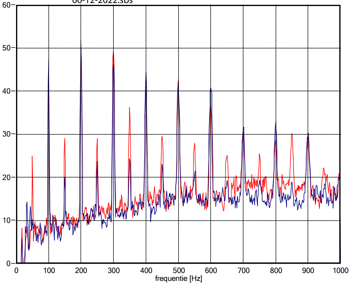
A-gewogen grafiek
