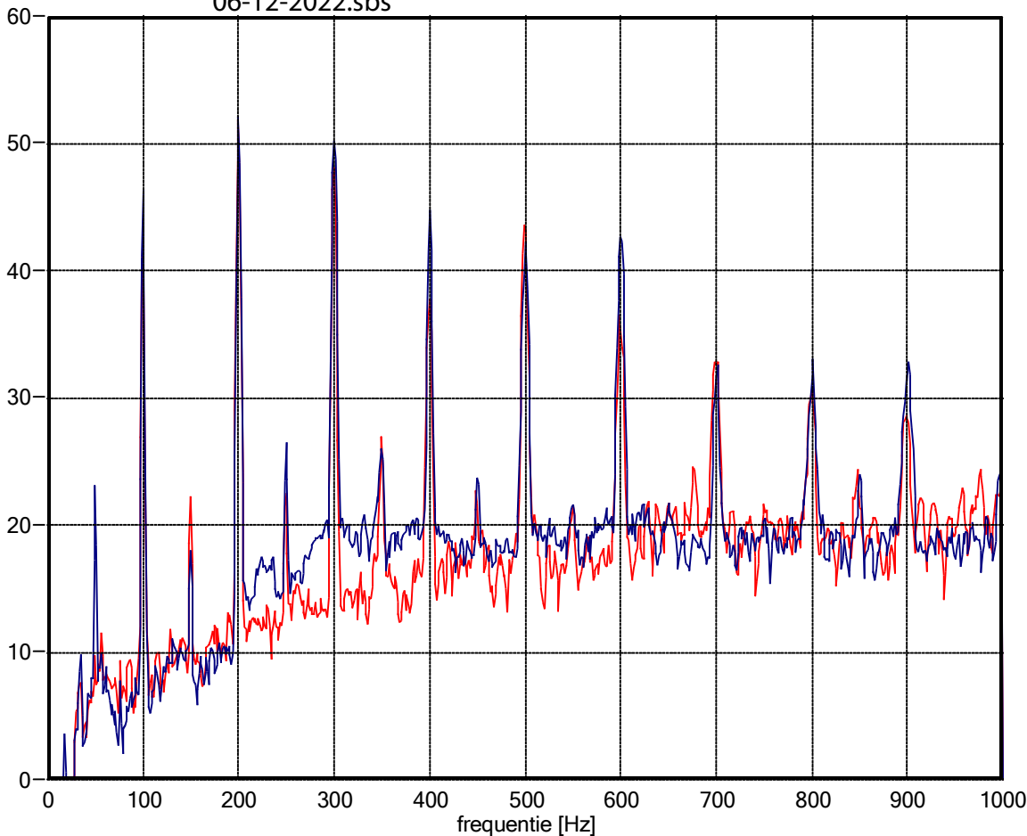
A-gewogen grafiek
