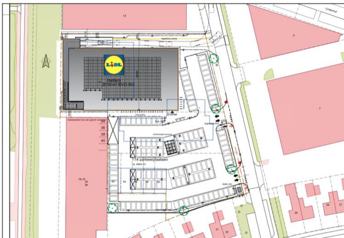
Afbeelding 3.1 Impressie plattegrond gewenste situatie (Bron: Bureau Korfker)
