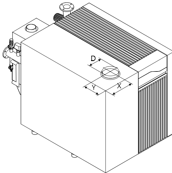
Fig. 19 Aansluiting luchttoevoer
