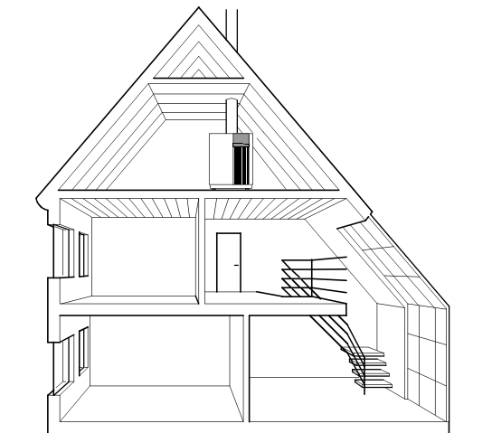
Fig. 15 Zolderopstelling
