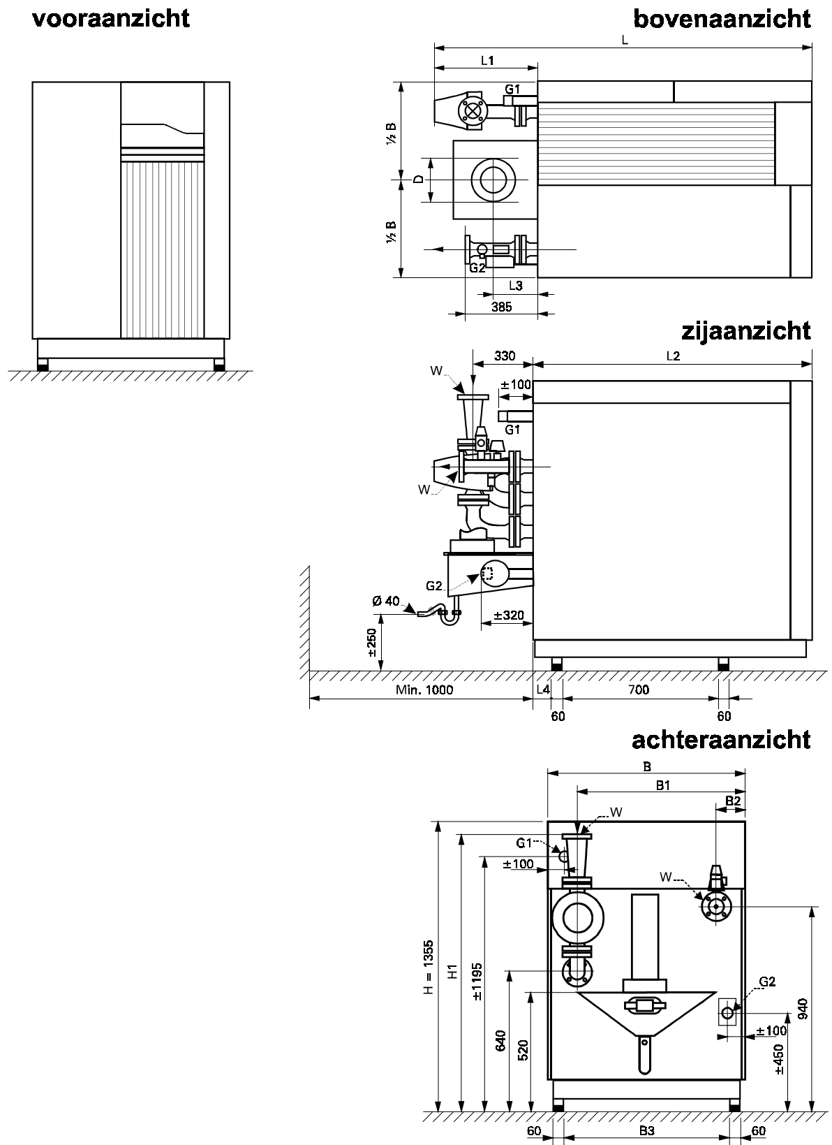
Fig. 2 Maatschets R2800
