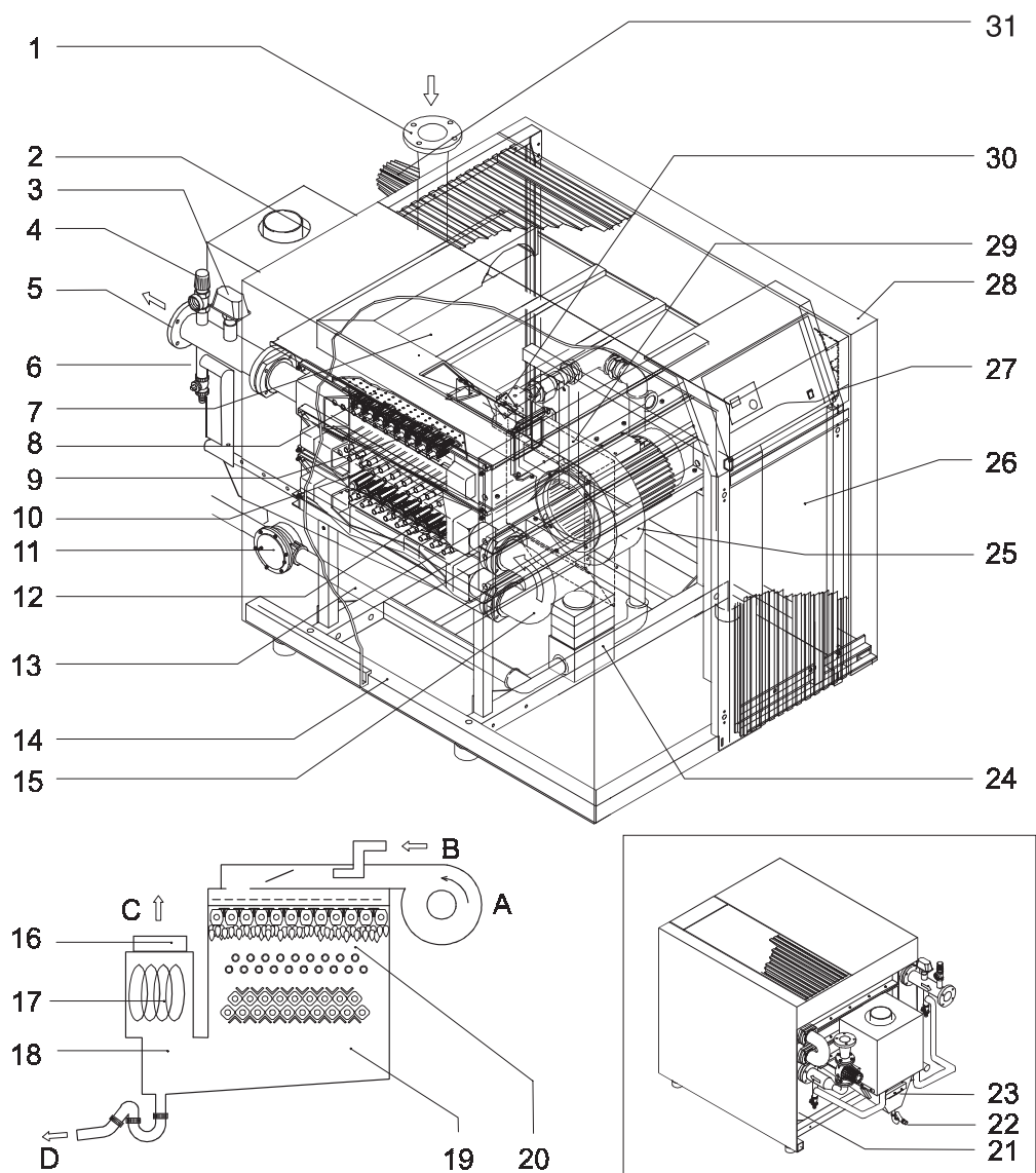
Fig. 5 Algemeen overzicht
