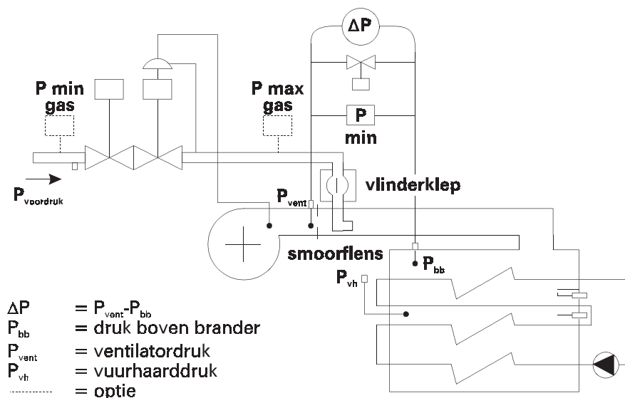
Fig. 36 Meten branderdruk
