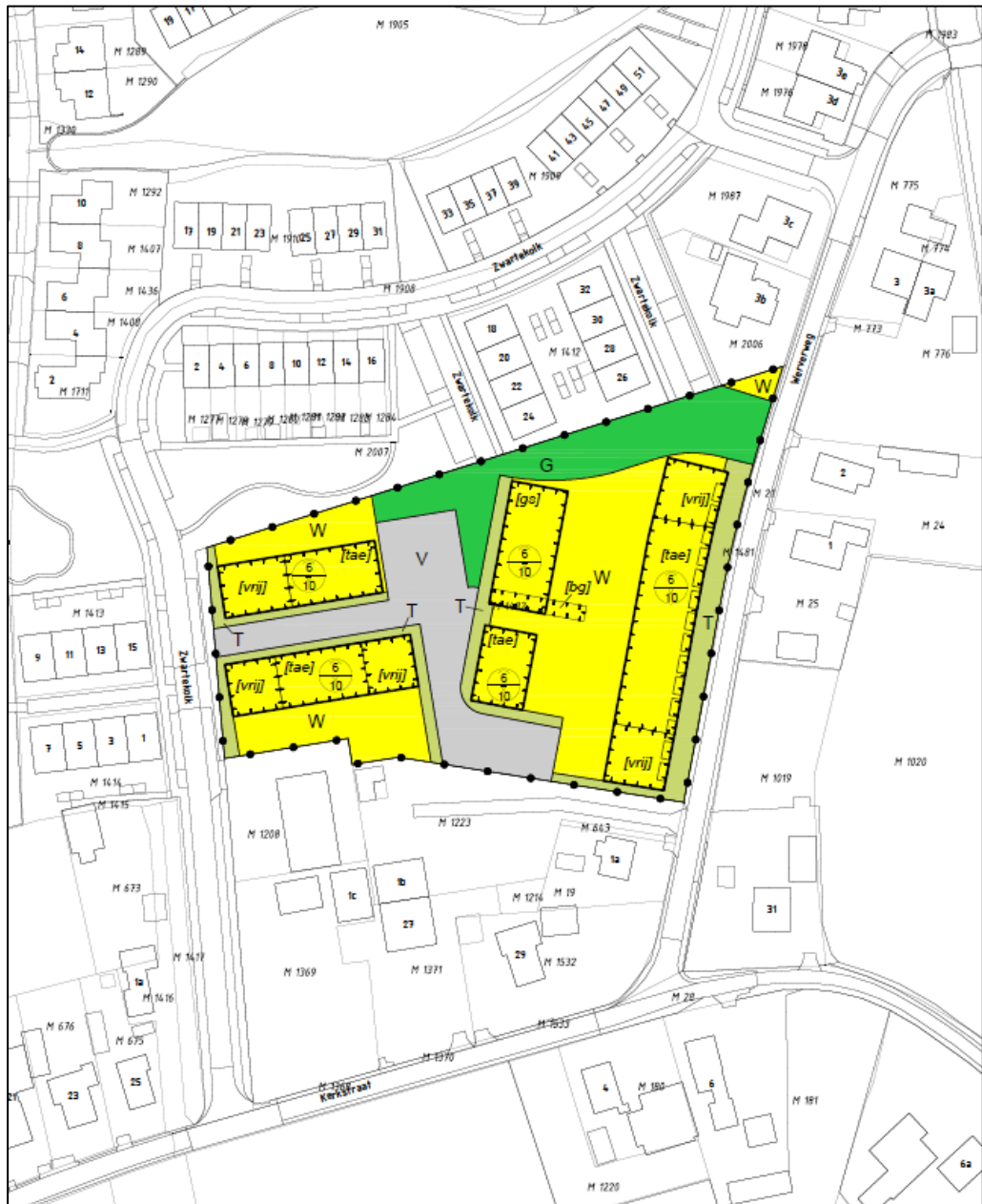
Planopzet woningbouwontwikkeling Zwartekolk/Werverweg te Wapenveld (d.d. 22-08-2023)
