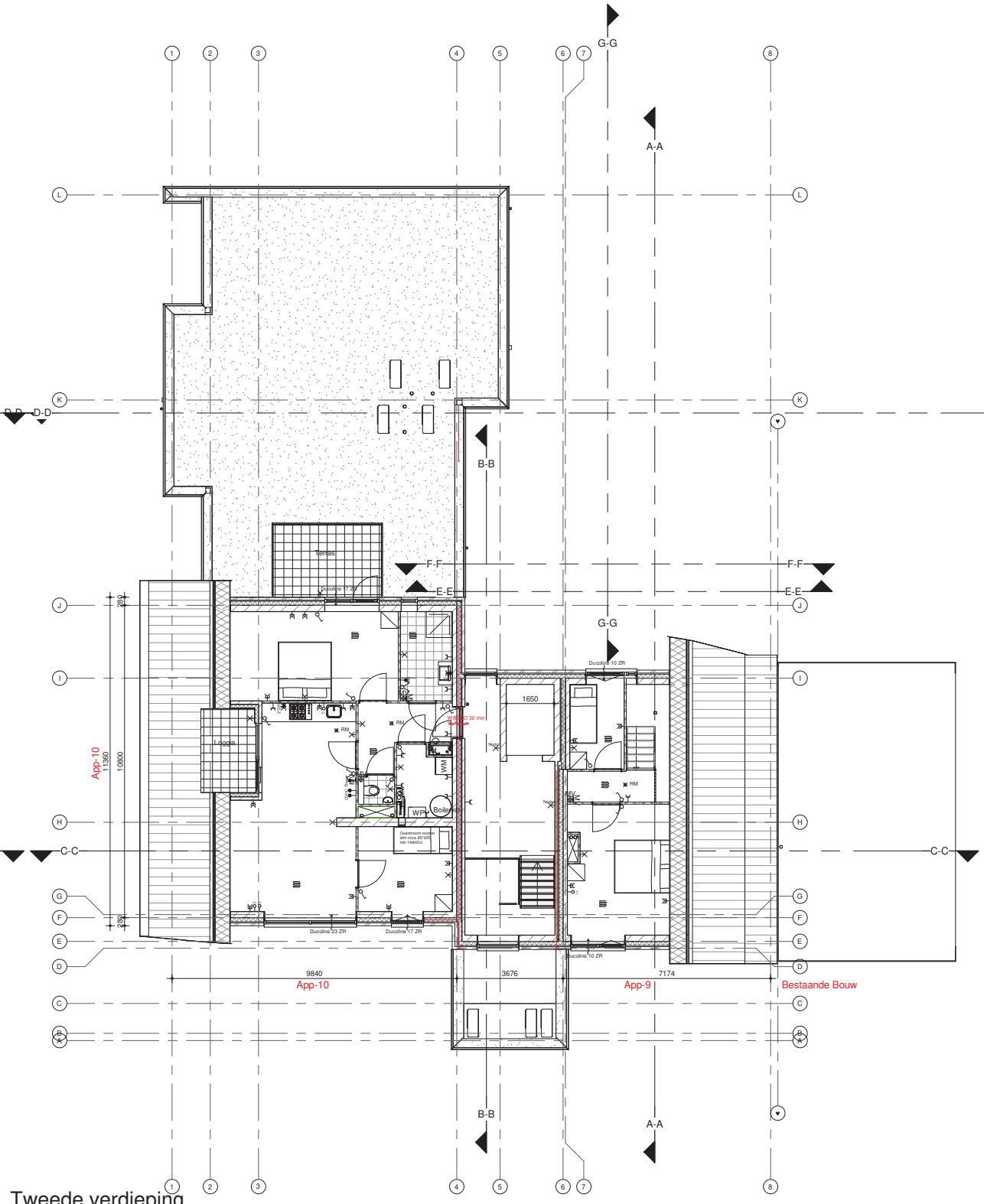
Tweede verdieping 1 : 100
