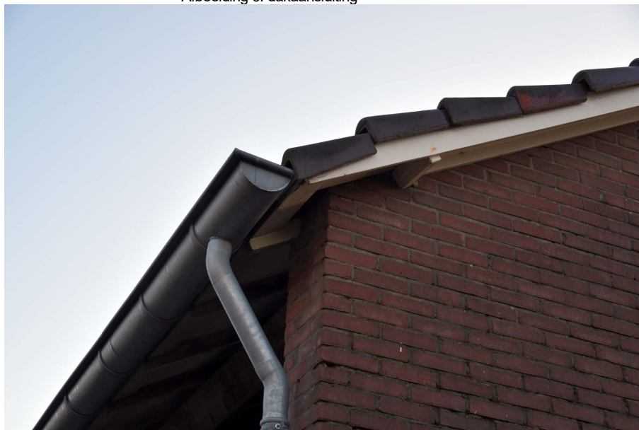
• Afbeelding 6: dakaansluiting
