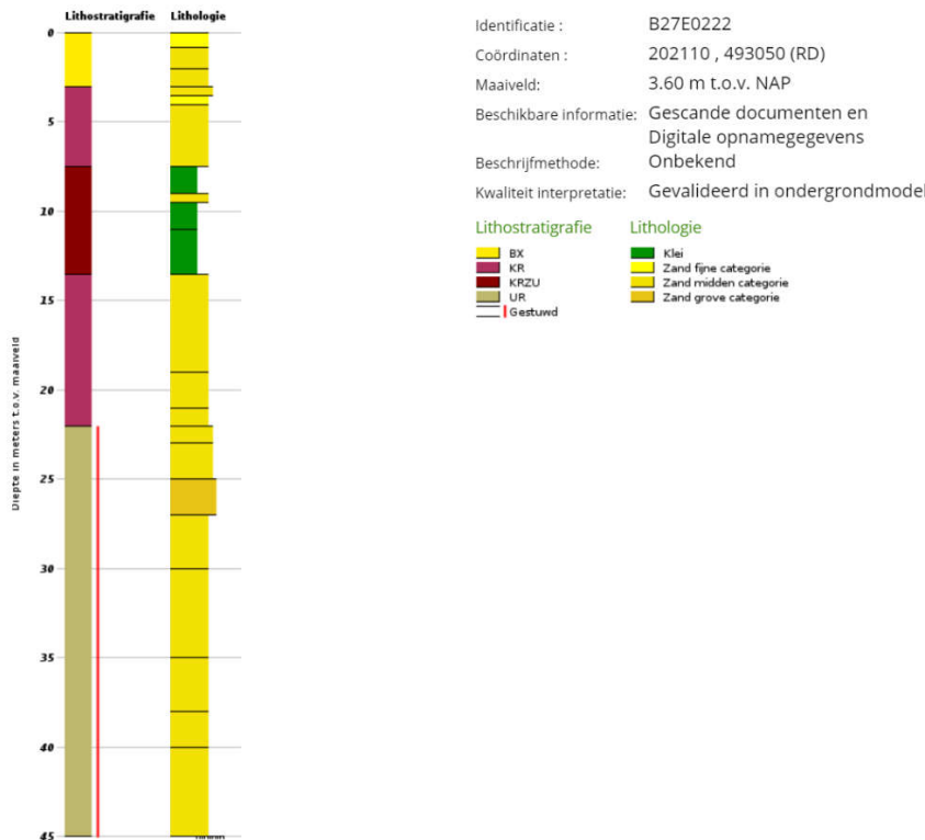
Boorbeschrijving boring B27E0222 (Dinoloket)
