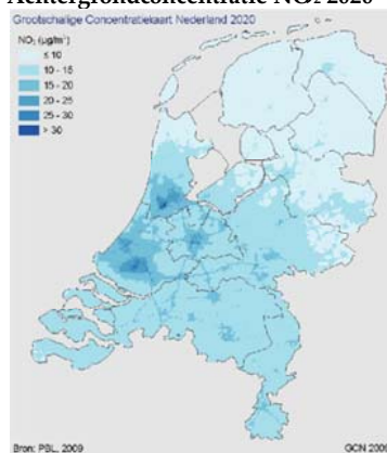
Achtergrondconcentratie NO 2 2020
