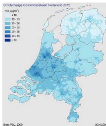
Achtergrondconcentratie NO 2 2015
