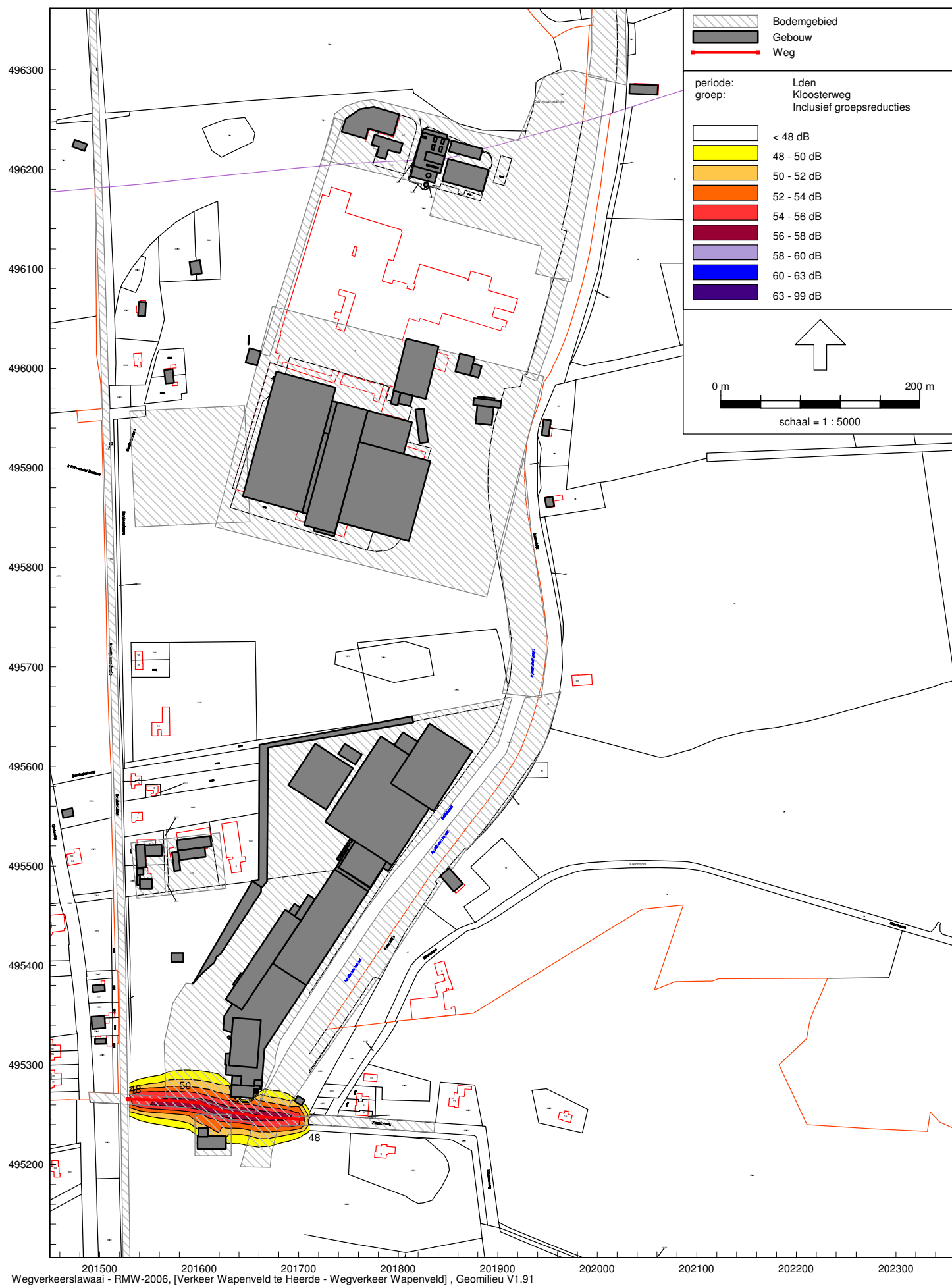
Geluidcontouren Kloosterweg met aftrek art. 110g Wgh Waarneemhoogte is 5 meter
