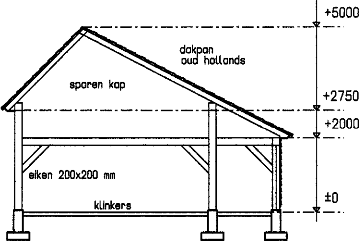
Doorsnede
