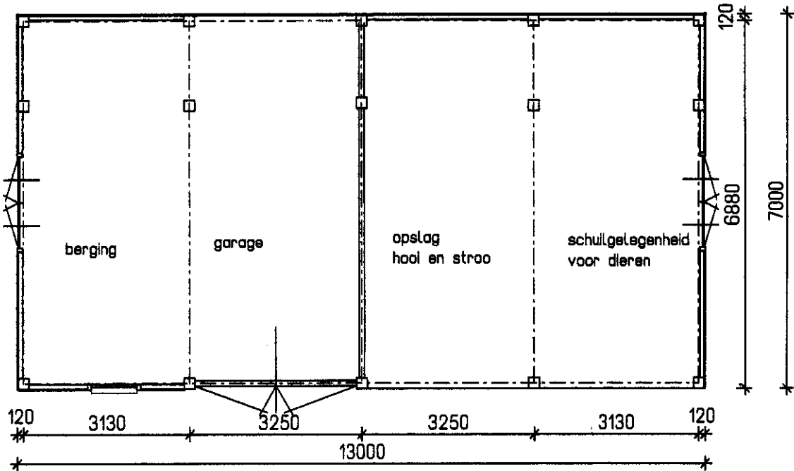
Plattegrond
