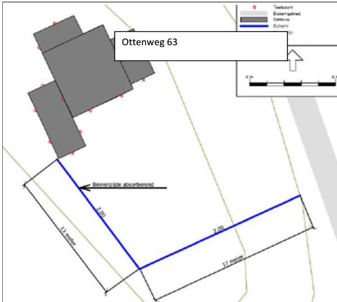
Figuur 3. Impressie van de plannen van het geluidsscherm aan de Ottenweg 61 en 63 te Oldebroek.
