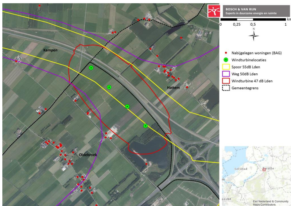
Figuur 8: Geluidscontouren van drie geluidsbronnen: windturbines, wegverkeer en spoorwegverkeer. 5
