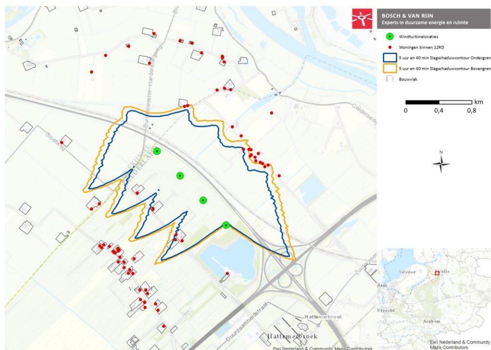
Figuur 9: slagschaduw onder- en bovengrens.
