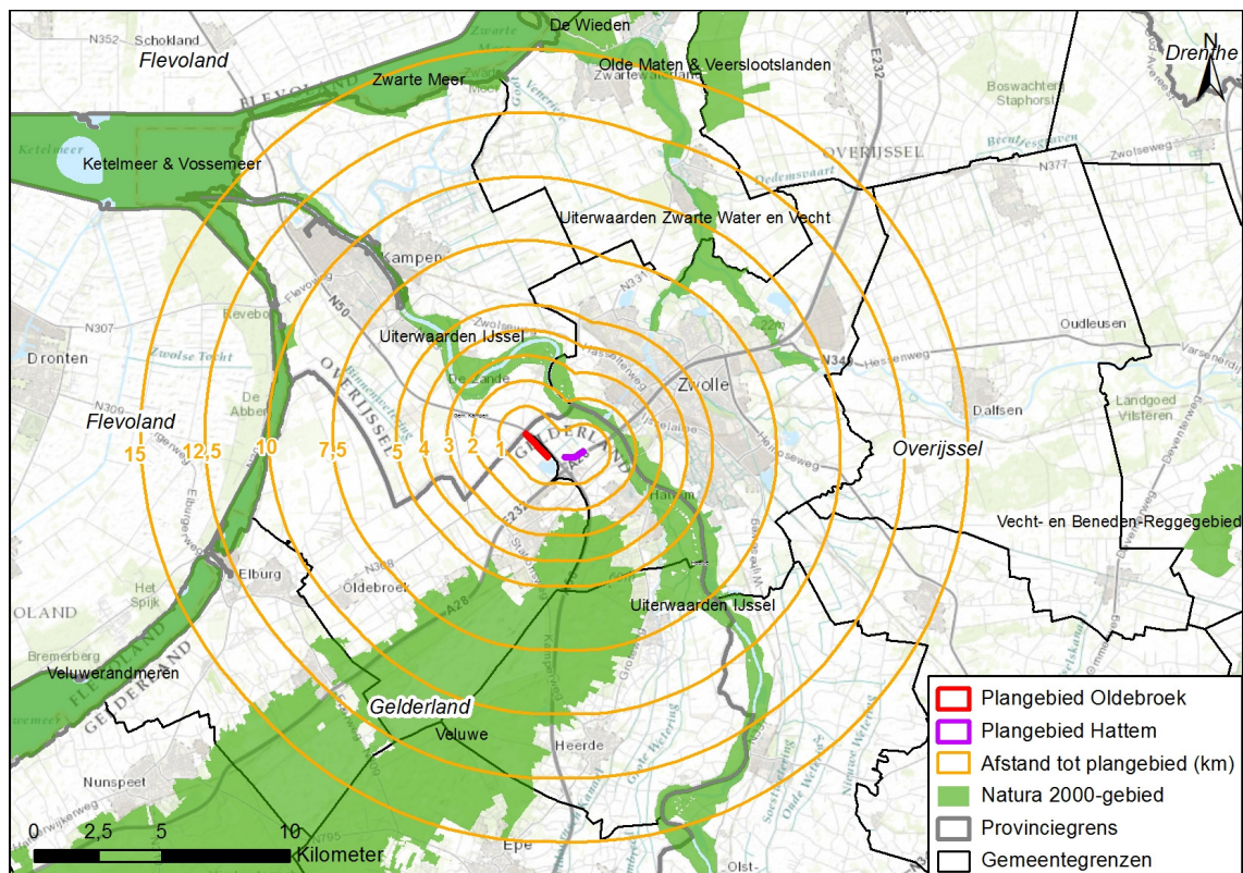
Figuur 4.1. Natura 2000-gebieden binnen 15 km van het plangebied. Bron: gebiedendatabase Ministerie van Economische Zaken
