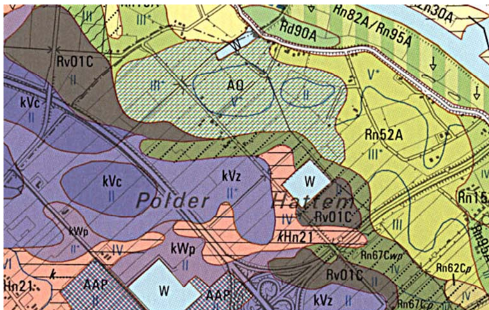
Figuur 2. Uitsnede bodemkaart van Nederland, blad 21 West Zvolle
