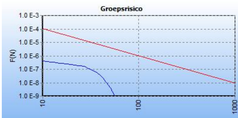
5.5 Figuur 5.5 FN curve voor N-570-21 van N.V. Nederlandse Gasunie voor de kilometer tussen stationing 0.00 en stationing 1000.00
