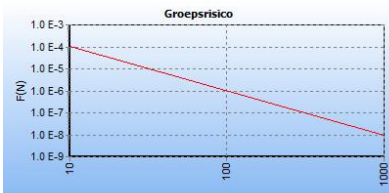
5.8 Figuur 5.8 FN curve voor N-570-37 van N.V. Nederlandse Gasunie voor de kilometer tussen stationing 0.00 en stationing 170.00
