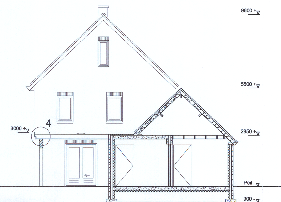
Doorsnede B-B
