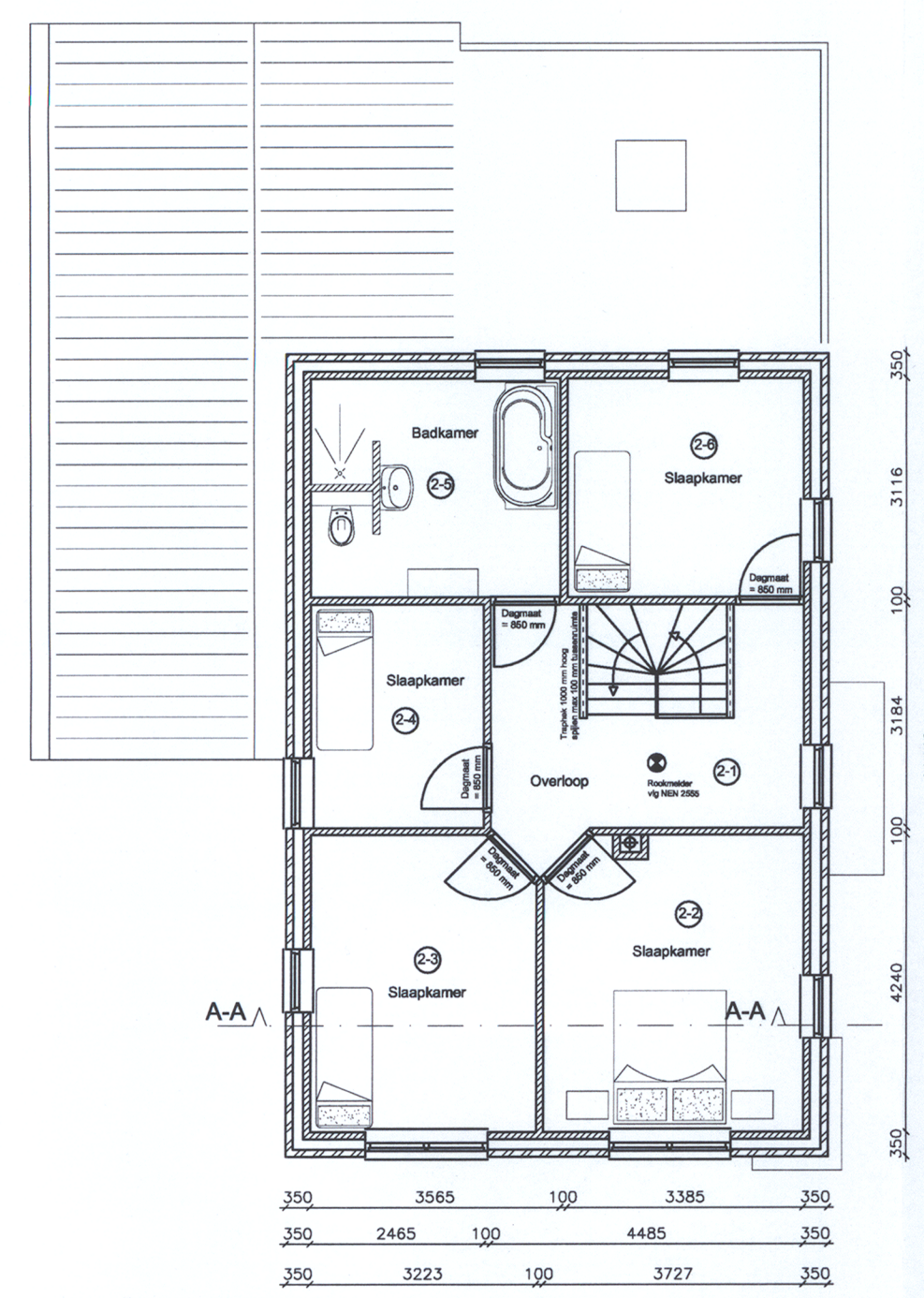
Verdieping
