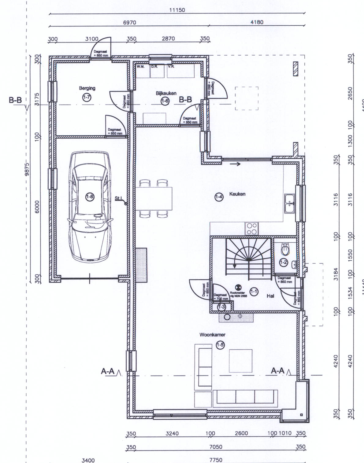
Begane grond
