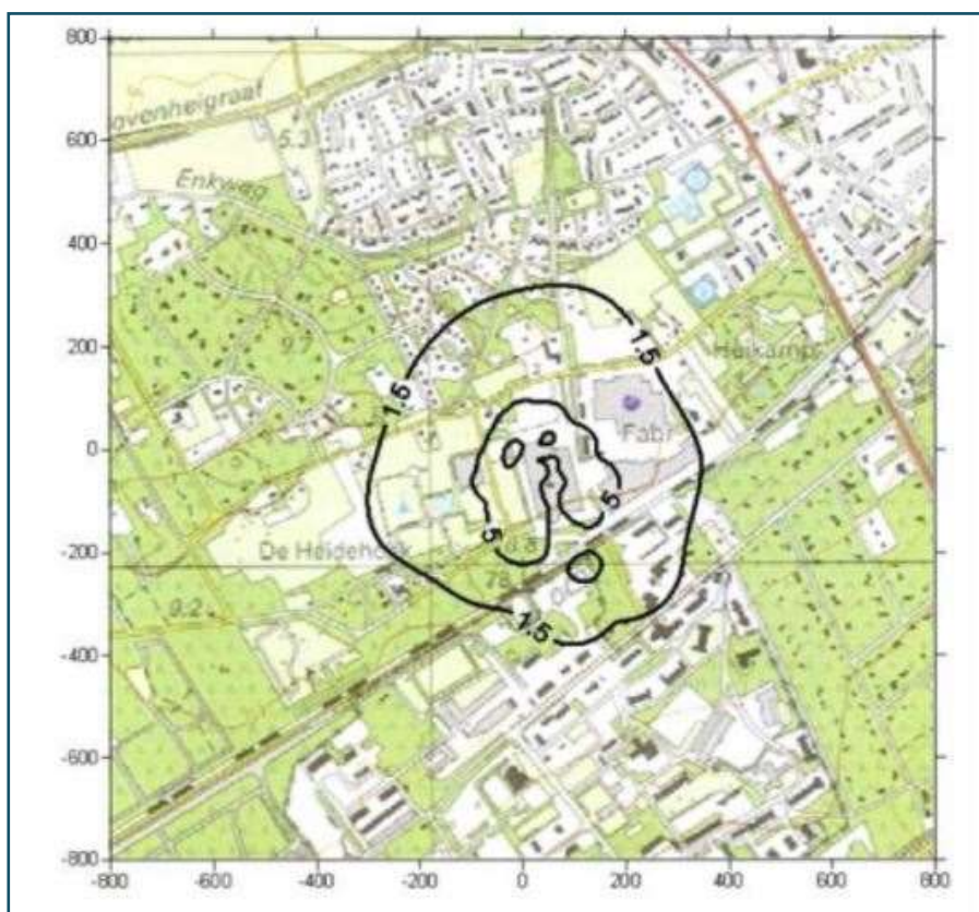
Figuur 3 Geurcontour voor vergunde productiecapaciteit van 100.000 ton per jaar
