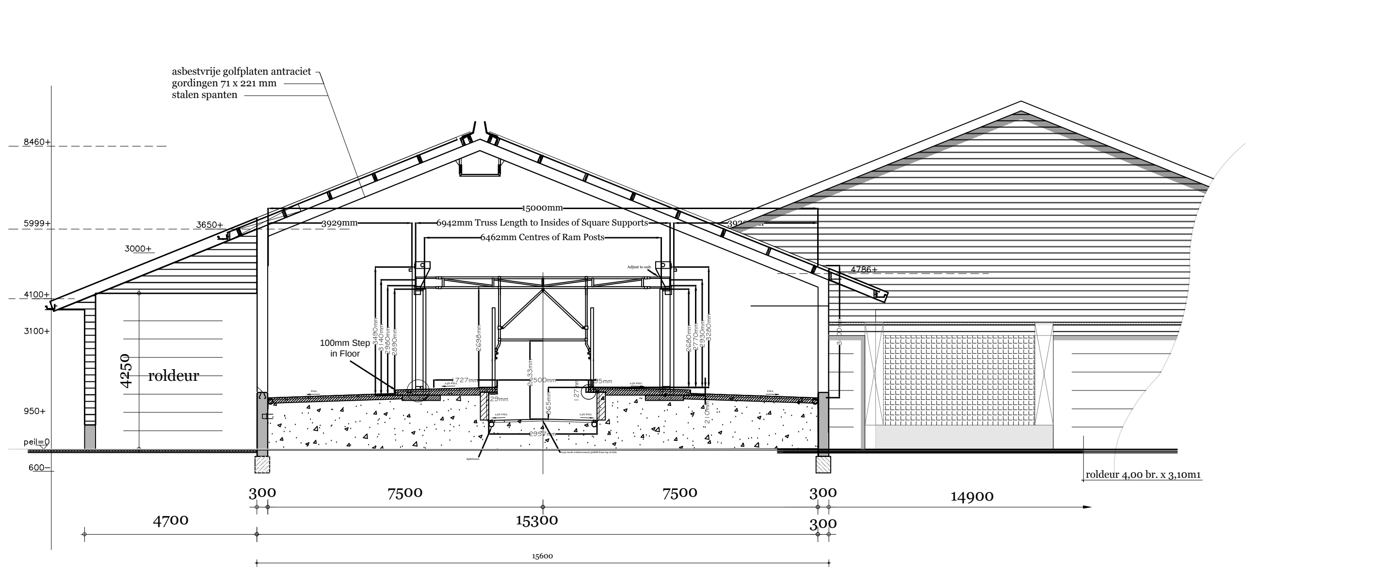
doorsnede A
