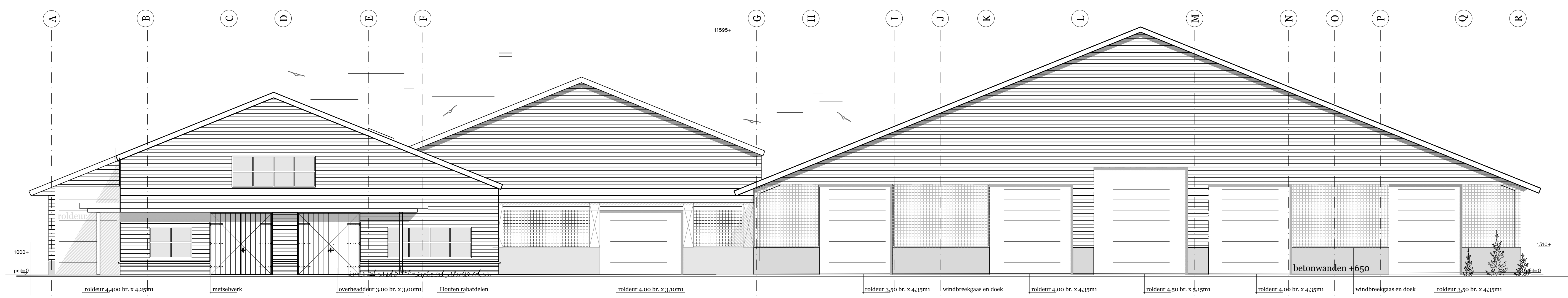
gevelaanzicht As 29
