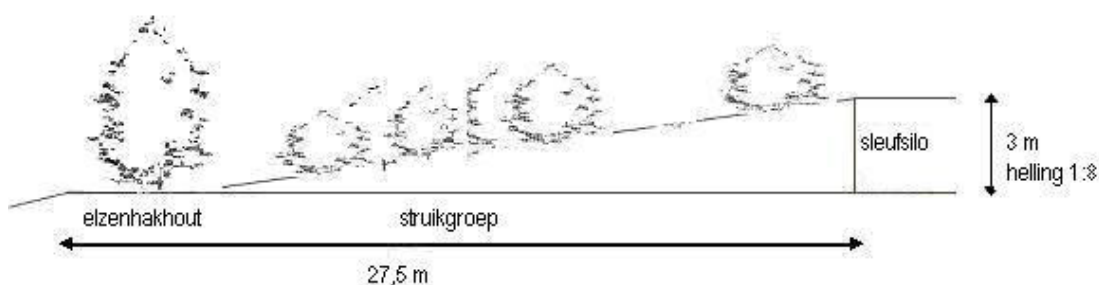
Dwarsdoorsnede A-B: gronddijk langs sleufsilo
