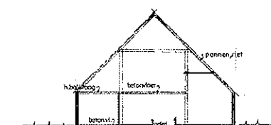
doorsnede C-C
