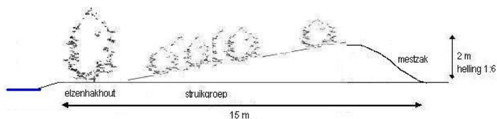
Dwarsdoorsnede A-A: gronddijk langs mestzak
