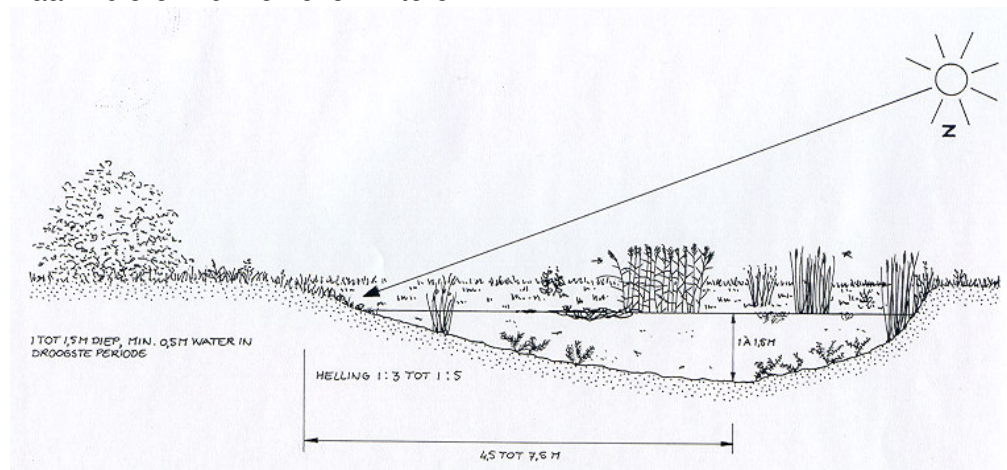
Tekening 2. Doorsnede poel
