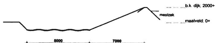
Dwarsdoorsnede A-A
