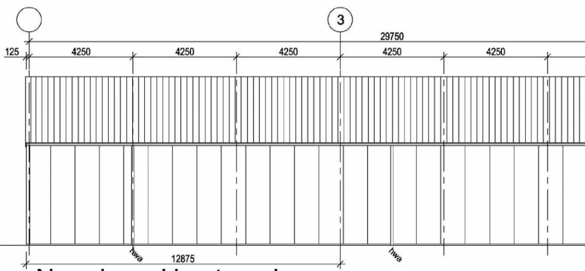
Noordgevel bestaand
