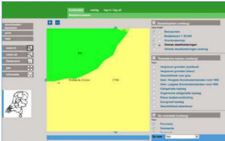
figuur 12: grondwatertrap (bron: Bodemdata)
