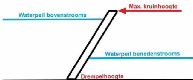
Figuur 11: Zijaanzicht stuw
