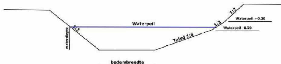
Figuur 9: Profiel natuurvriendelijke oever
