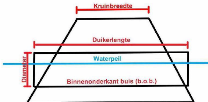
Figuur 10: Zijaanzicht duiker
