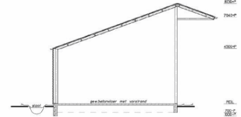
hoogtedoorsnede
