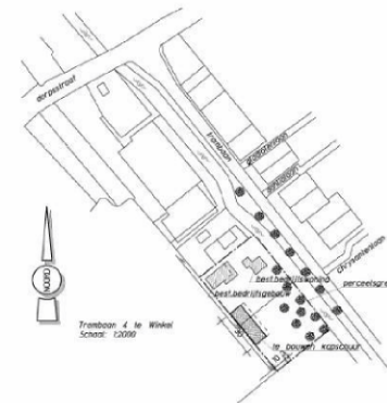
situatie
