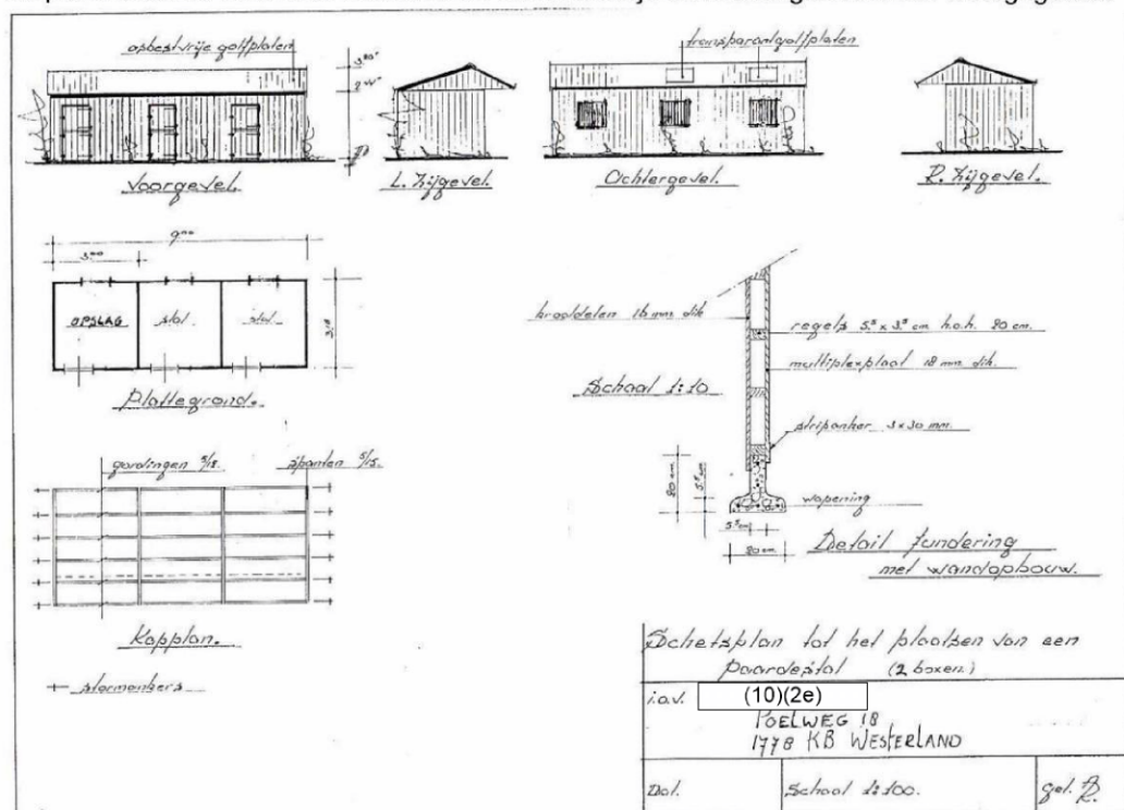
Bouwtekeningen paardenstal
