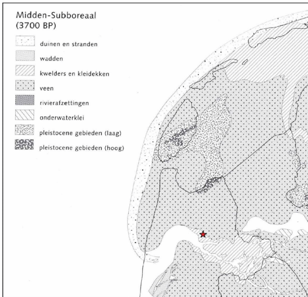
Abbeelding I Paleogeografische situatie rond 3700 BP; planlocatie weergegeven met ster. (bron: Zagwijn 1986)
