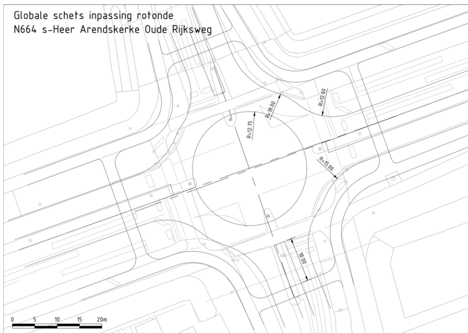
Afbeelding 3.6: globaal ruimtebeslag rotonde
