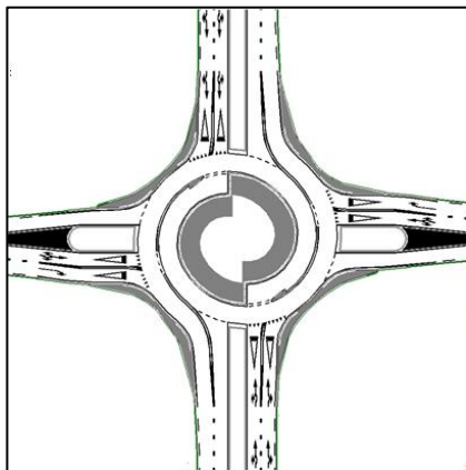
Afbeelding 3.4: minimaal gewenste vormgeving turborotonde op deze locatie
