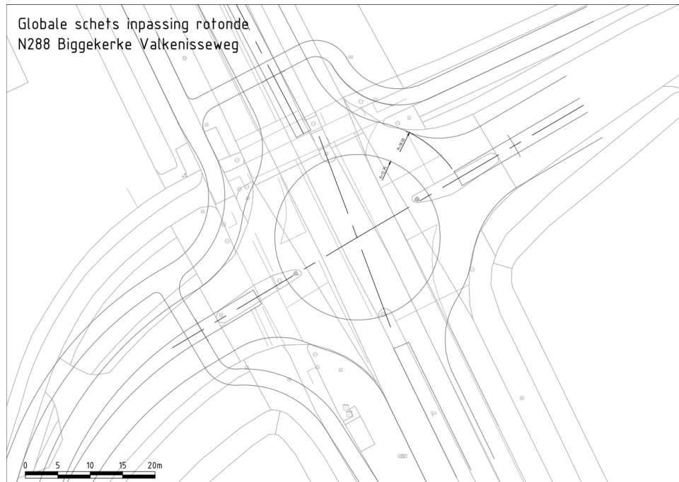
Afbeelding 3.2: globaal ruimtebeslag rotonde
