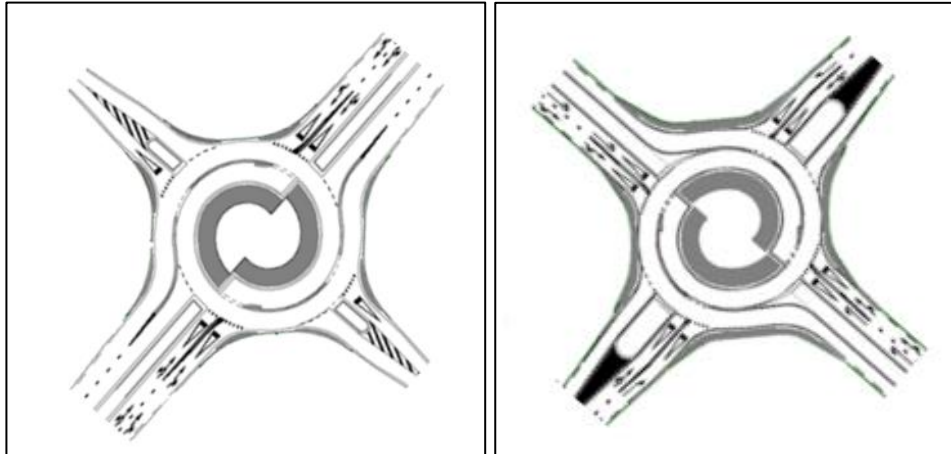
Afbeelding 3.22 rijstrookindeling eirotonde (links) en partiële turborotonde (rechts)
