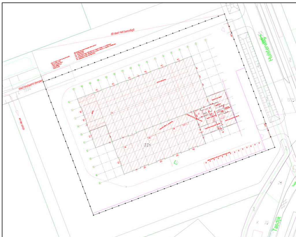
Schetsontwerp met plattegrond voorlopige indeling bedrijfsp perceel.
