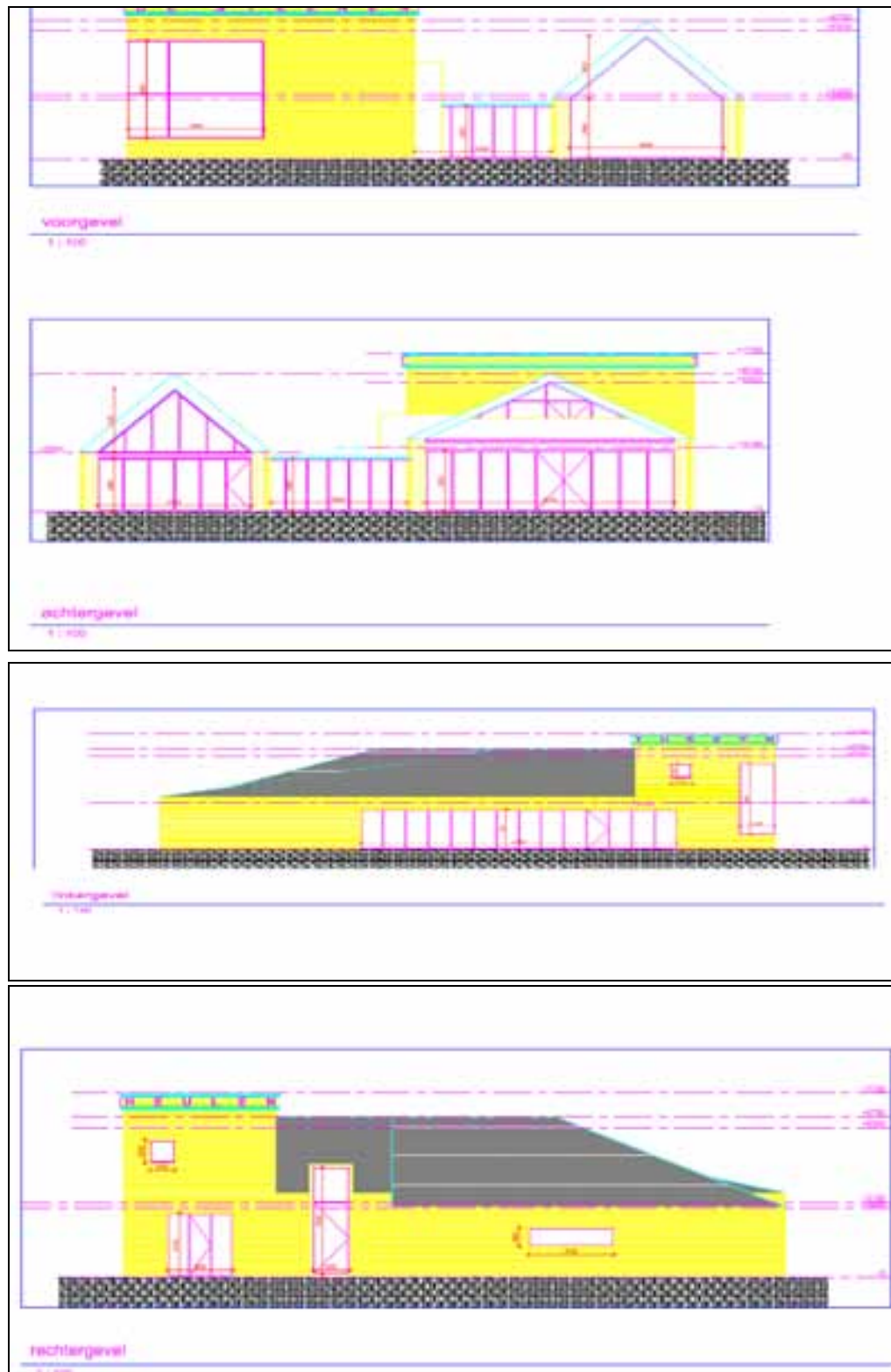
Figuur 5 gevelaanzichten bouwplan
