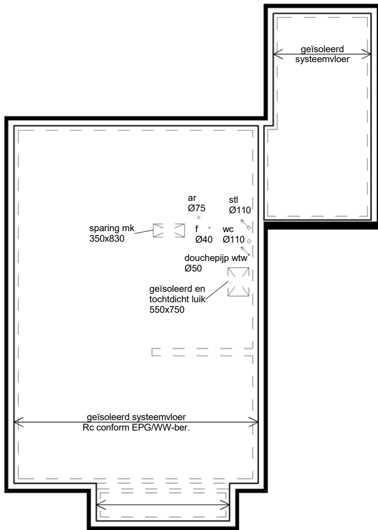
begane grondvloer
