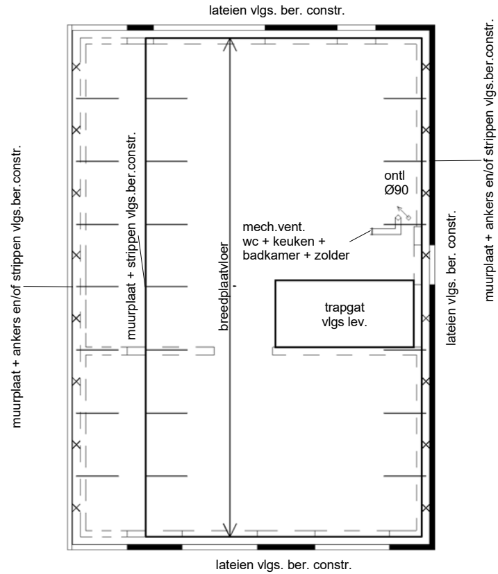
zoldervloer
