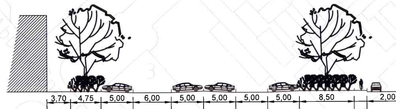
DWARSDOORSNEDE A-A
