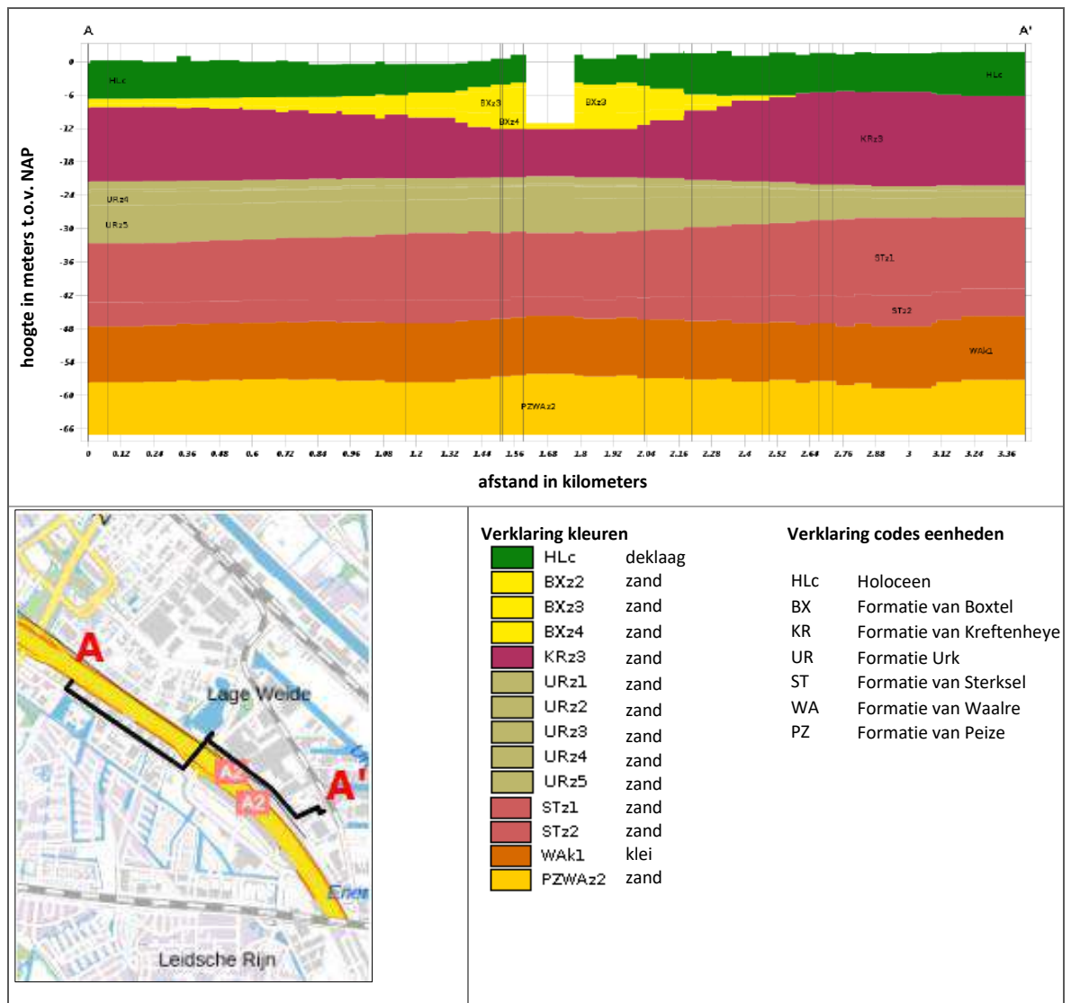
Figuur 3.3: hydrogeologische bodemopbouw S6227-S6265 Utrecht (bron: Dino-loket, REGIS II.2)
