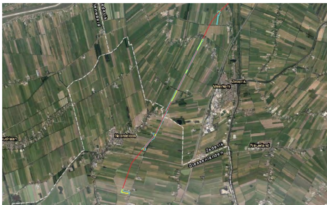
Figuur 4.14. Het zuidelijke deel van het HTL tracé. De HDD-borings zijn in rood weergegeven, geel betreffen open ontgravingen. De werkstroken zijn blauw weergegeven (bron achtergrond: Esri).
