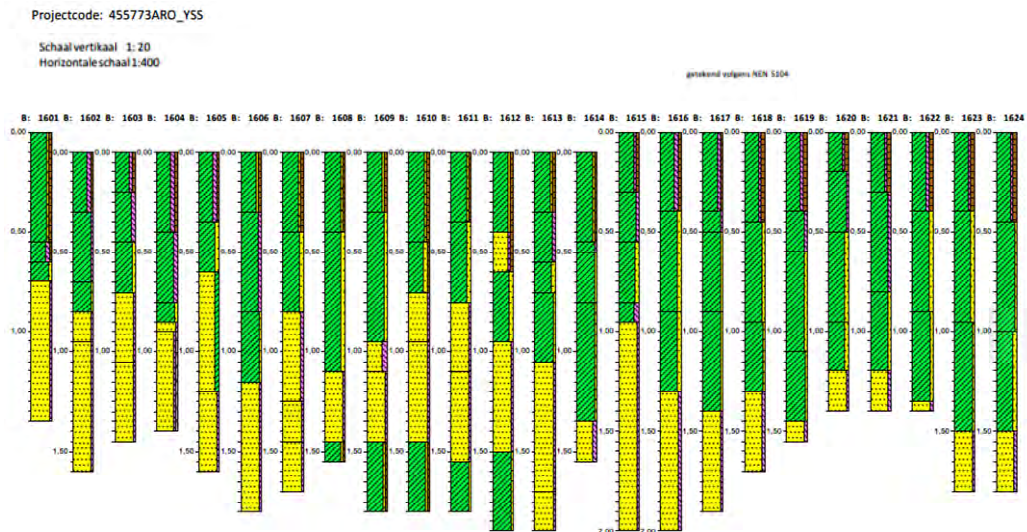
Afbeelding 15. Dwarsprofiel boringen 1601-1624.
