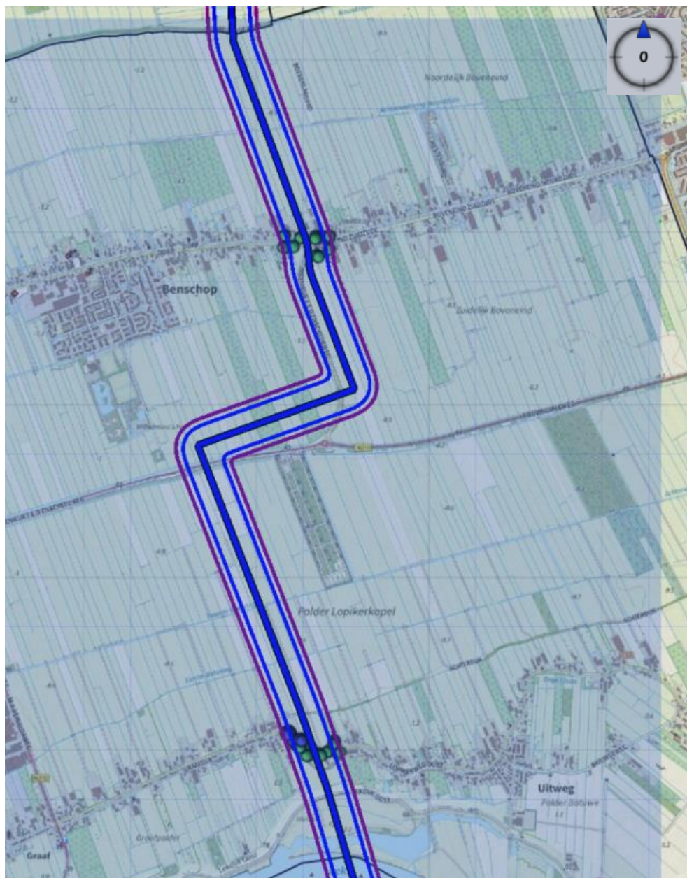
Figuur 13: Plaatsgebonden risico rondom aardgasleiding A-555-08 gemeente Lopik
