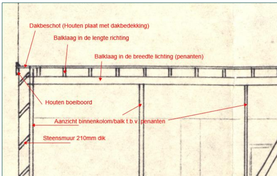
Figuur 3.1 Opbouw van de gevels en het dak waarbij het ontbreken van een spouw en dakruimte zichtbaar zijn.
