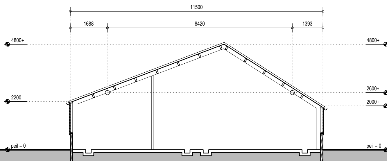
doorsnede: B
