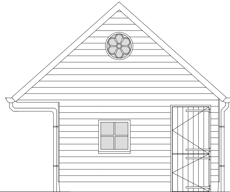
ACHTERGEVEL
