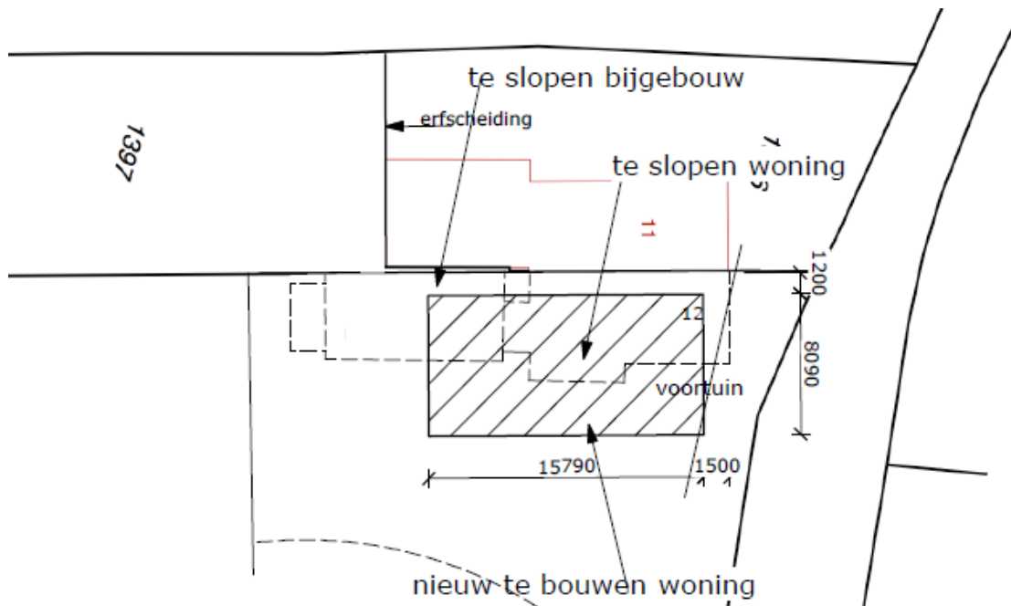
Situatietekening toekomstige situatie (bron: Bureau van Beek)
