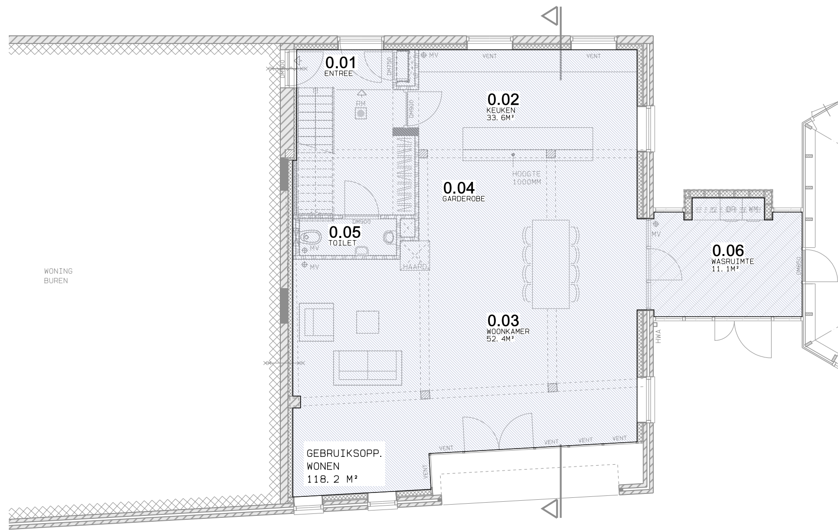
BEGANE GROND GEBRUIKSOPPERVLAKTE
