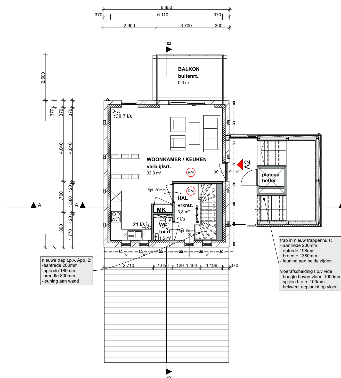
3e verdieping (gewijzigd)
