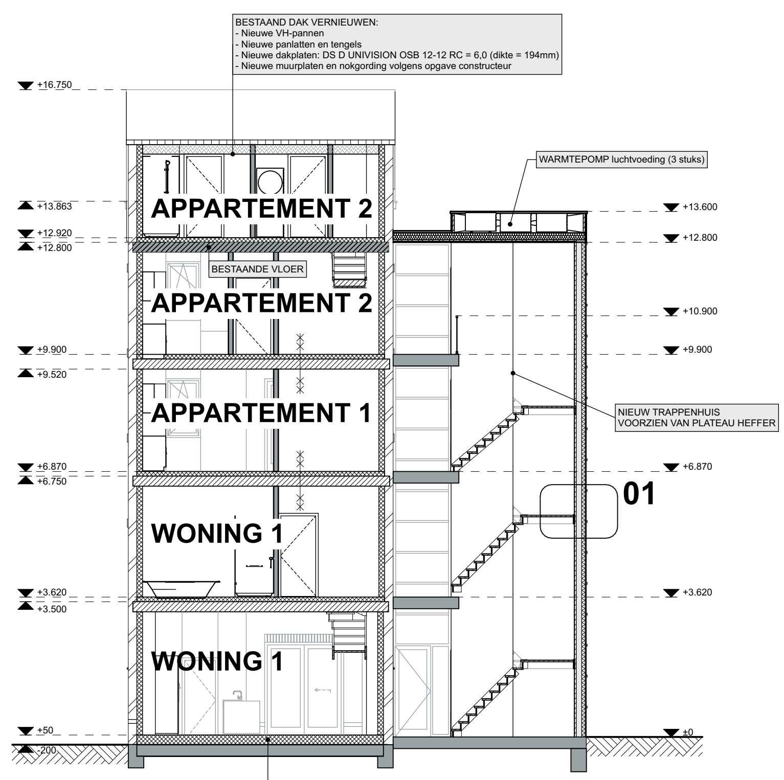
DOORSNEDE A-A (gewijzigd)
