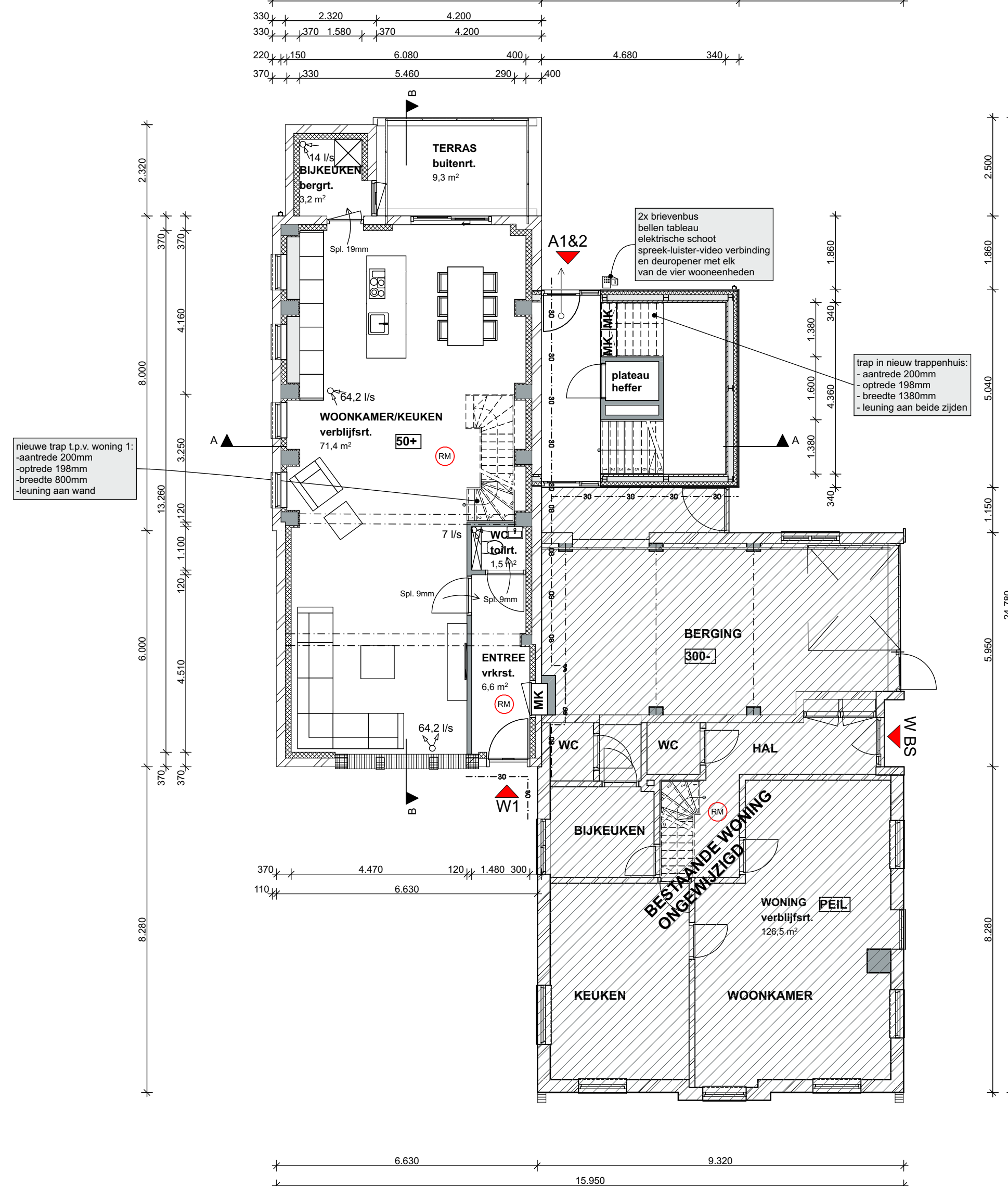
BEGANE GROND (gewijzigd)
