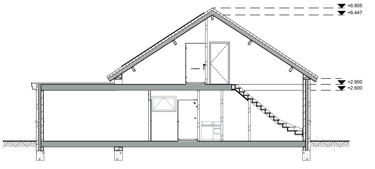
DOORSNEDE B-B
