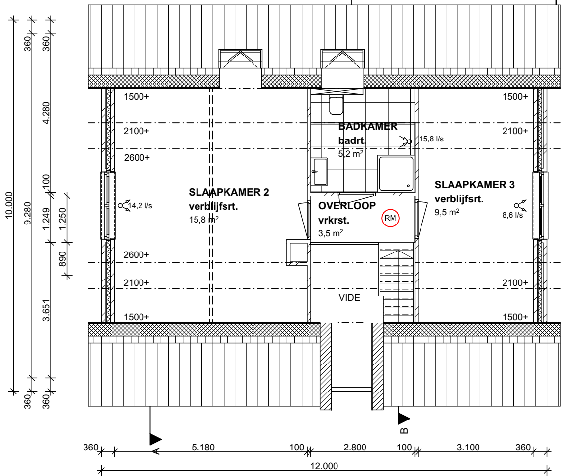
1e VERDIEPING
