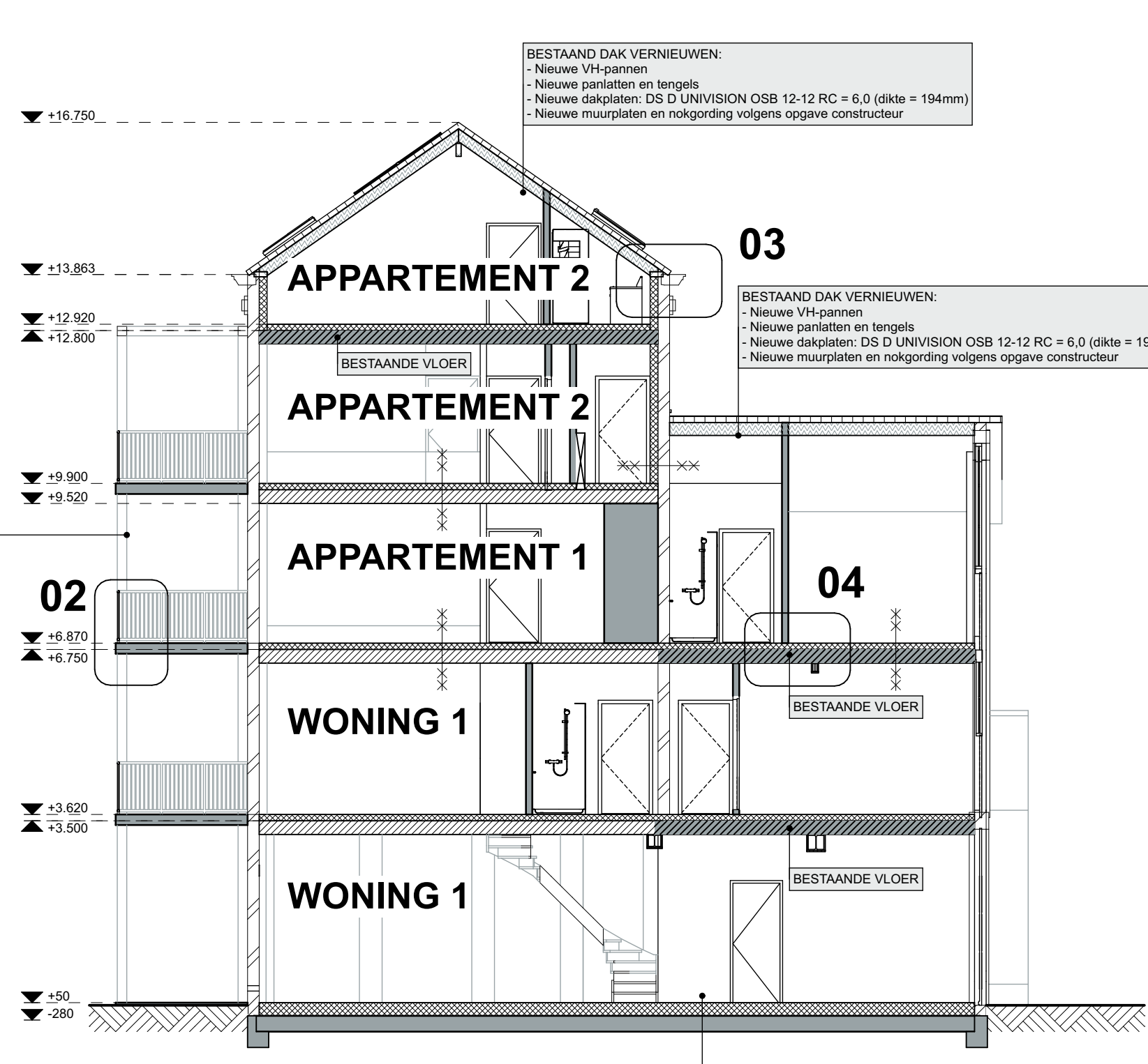
DOORSNEDE B-B (gewijzigd)
