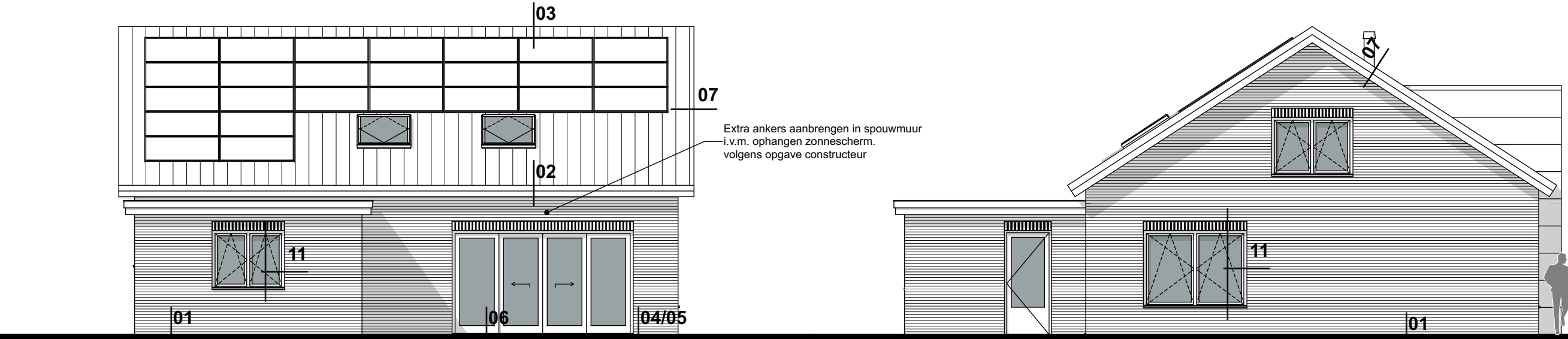
ACHTERGEVEL - ZUIDOOST
