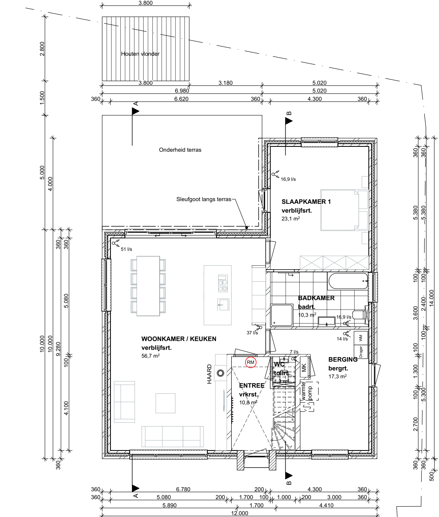
BEGANE GROND
