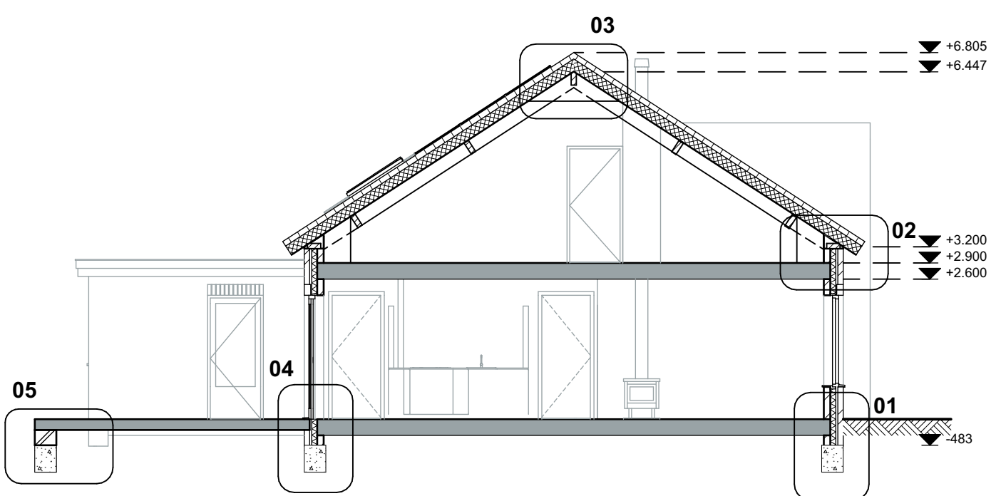
DOORSNEDE A-A
