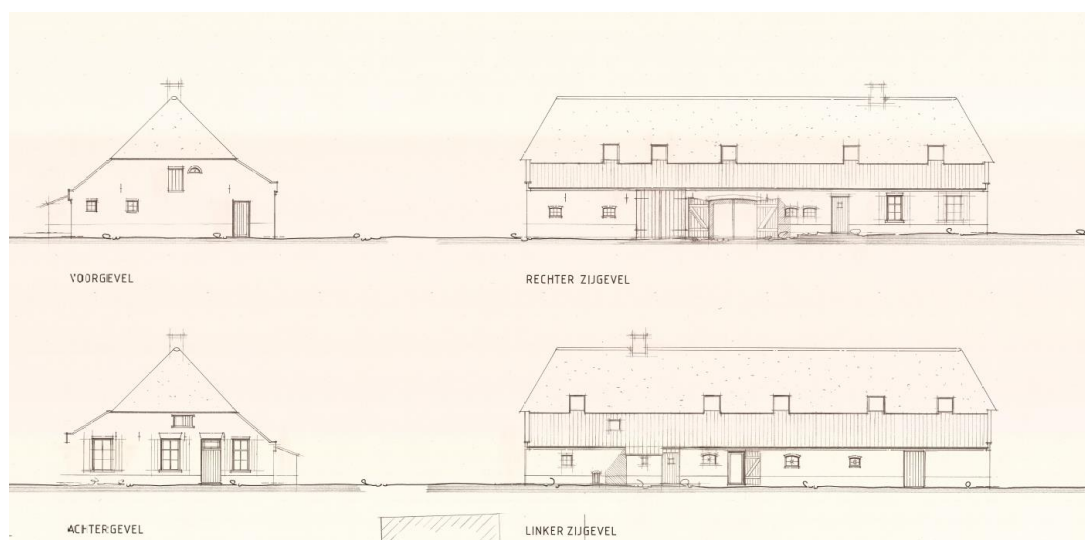
Beoogde situatie kortgevelboerderij
