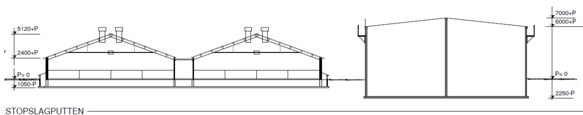
Figuur 6: doorsnede bestaande varkensstal en nieuw op te richten bebouwing
