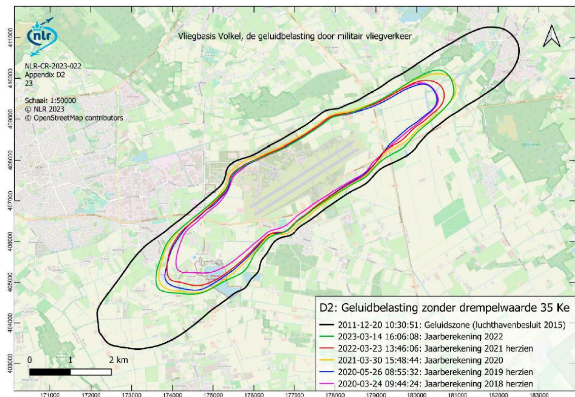
figuur 6 geluidsbelasting afgelopen 2018-2022 [9]
