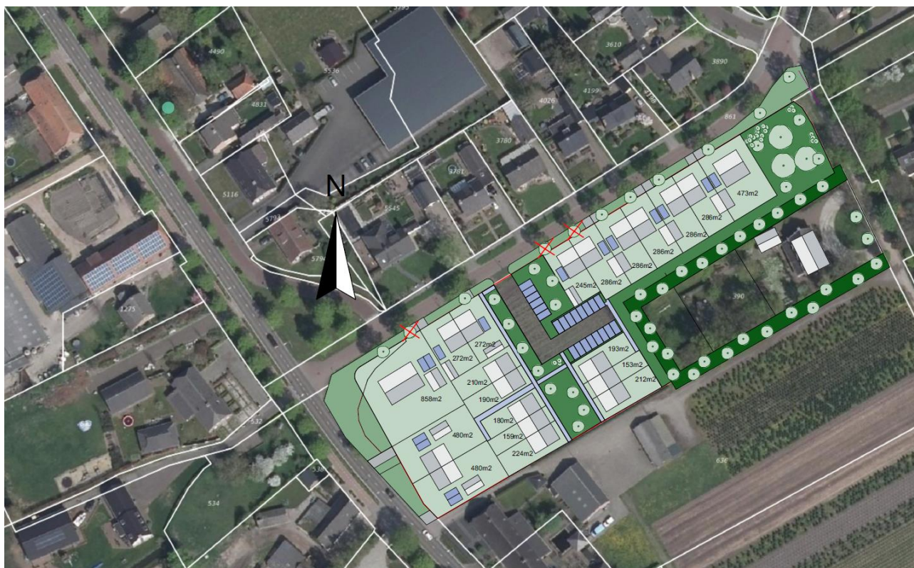
Figuur 3.1. Schets van de voorgestane situatie. Bron: LA | Architecten.
